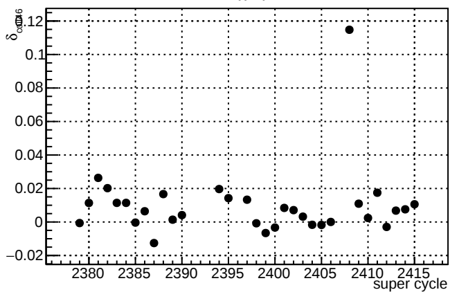
\delta_{\text{coil46}}
