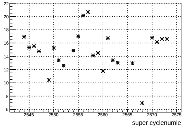
usl_4eY : slug 55
