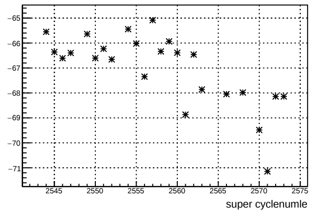
usl_4eY : slug 55
