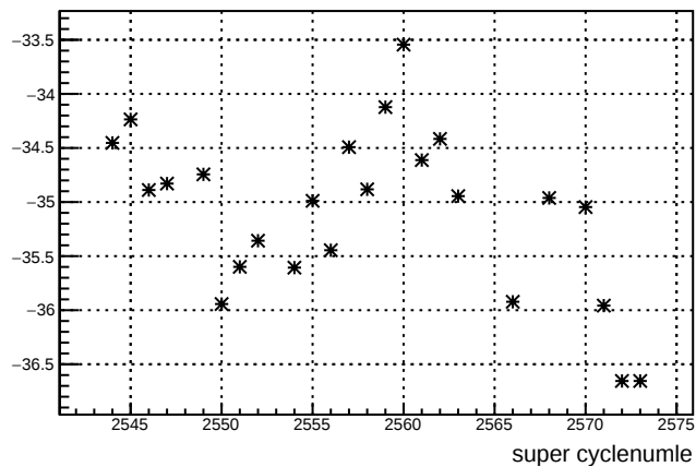
usl_11X12X : slug 55
