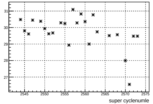
usr_4eY : slug 55
