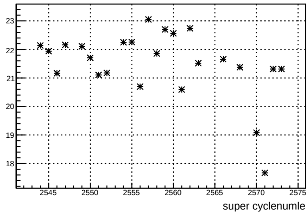
dsr_4eY : slug 55
