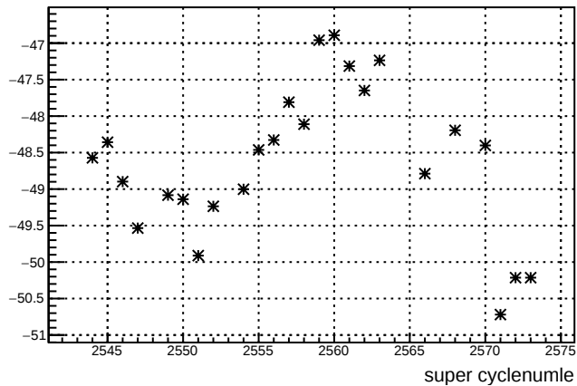
dsr_11X12X : slug 55
