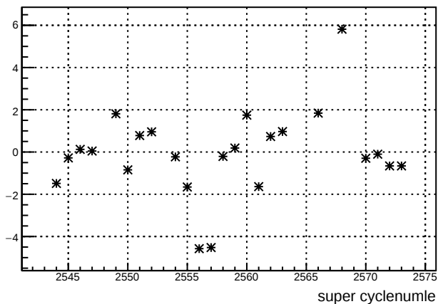
usl_11X12X : slug 55
