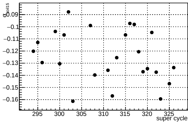
\alpha_{\text{coil15}}\text{--slug6}
