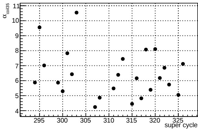
\alpha_{\text{coil35}}\text{--slug6}
