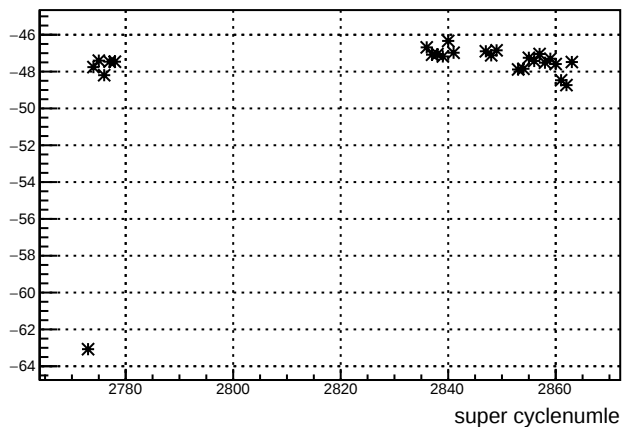
dsr_11X12X : slug 60
