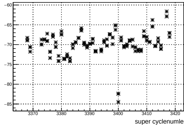
usl_4eY : slug 75
