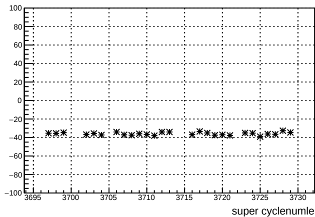
usl_11X12X : slug 83
