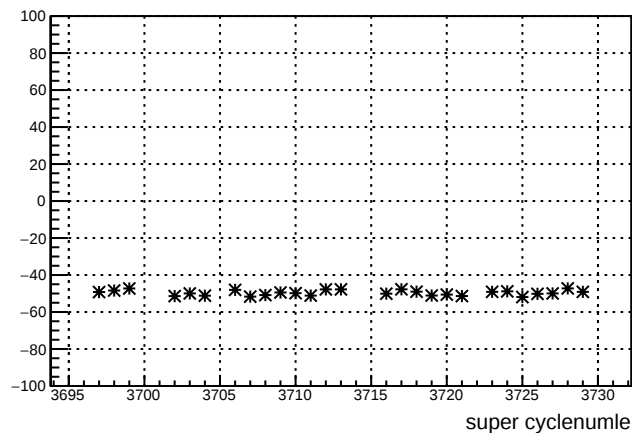
dsr_11X12X : slug 83
