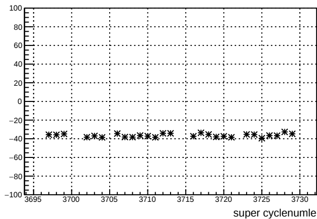
dsl_11X12X : slug 83
