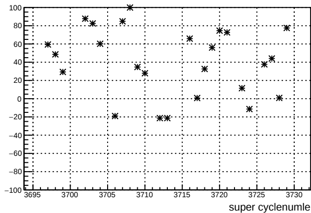
usl_4aY : slug 83
