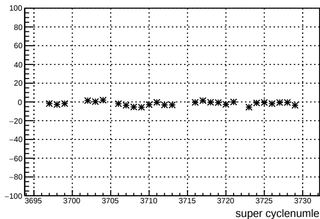
usl_11X12X : slug 83
