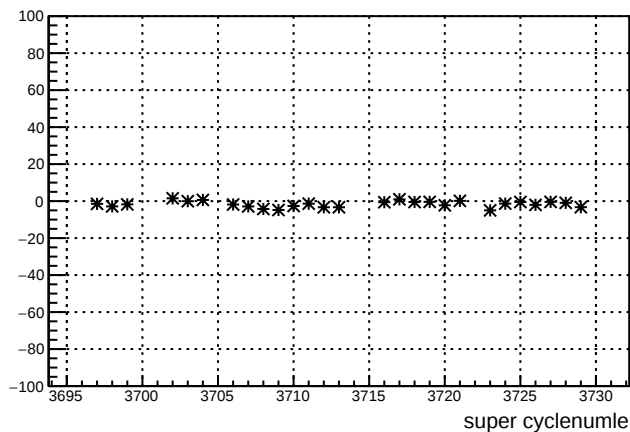
dsl_11X12X : slug 83
