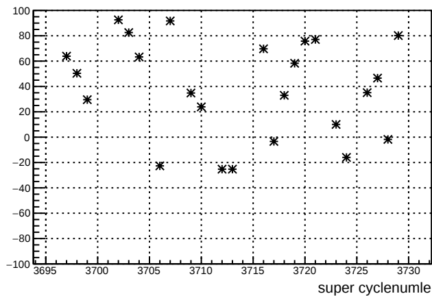
dsl_4aY : slug 83
