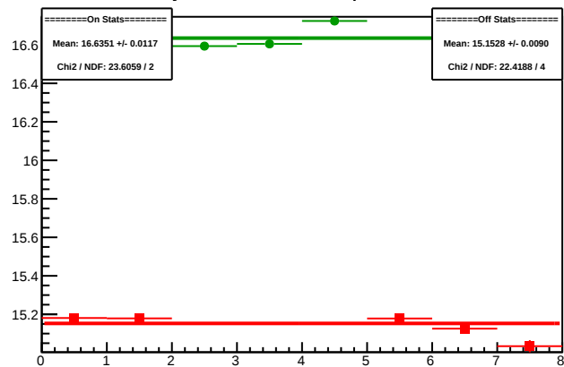
Cycle 4300.10: Multiplet Sums
