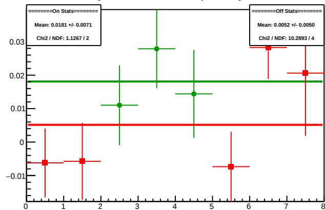
Cycle 4300.10: Multiplet Asyms
