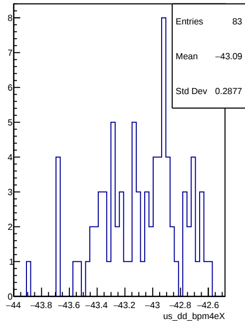
us_dd_bpm4eX
