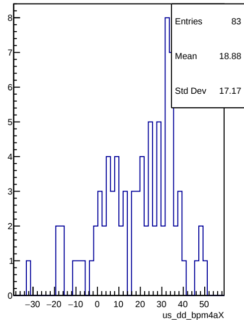
us_dd_bpm4aX
