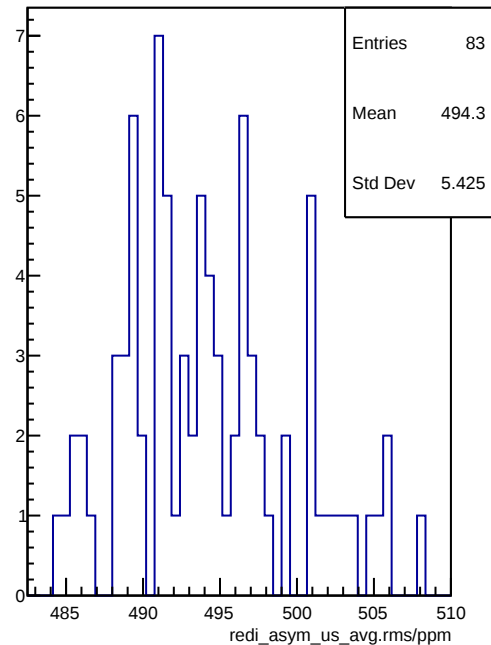
redi_asym_us_avg.rms/ppm
