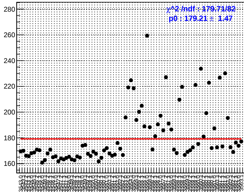
slug10: redi_asym_usl.rms/ppm
