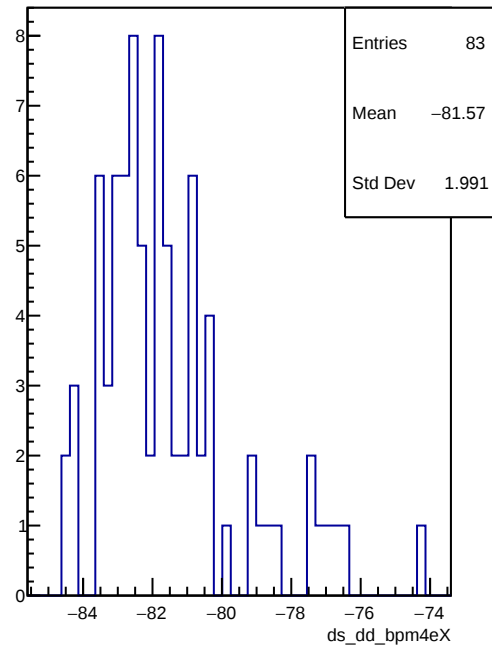
ds_dd_bpm4eX
