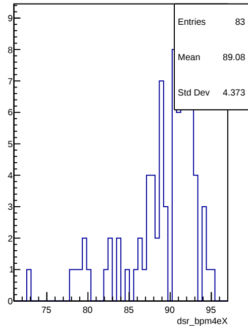
dsr_bpm4eX
