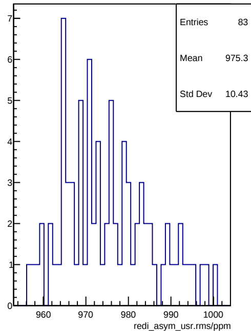
redi_asym_usr.rms/ppm
