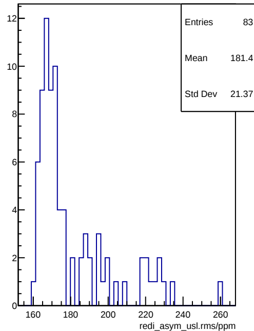
redi_asym_usl.rms/ppm
