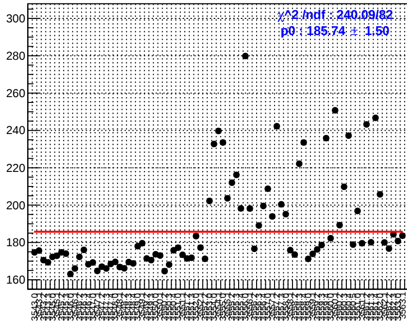
slug10: redi_asym_dsl.rms/ppm
