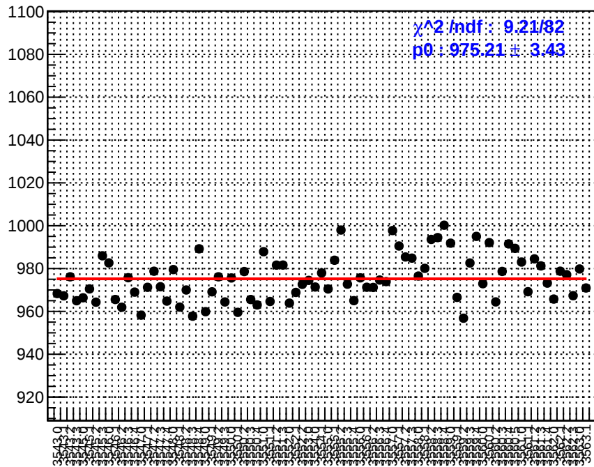
slug10: redi_asym_usr.rms/ppm
