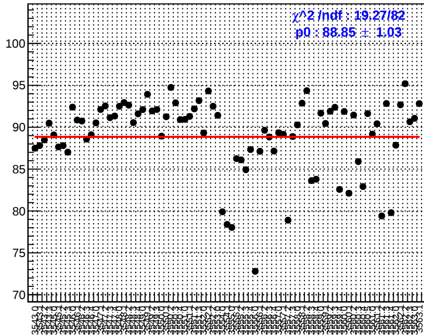
slug10: dsr_bpm4eX
