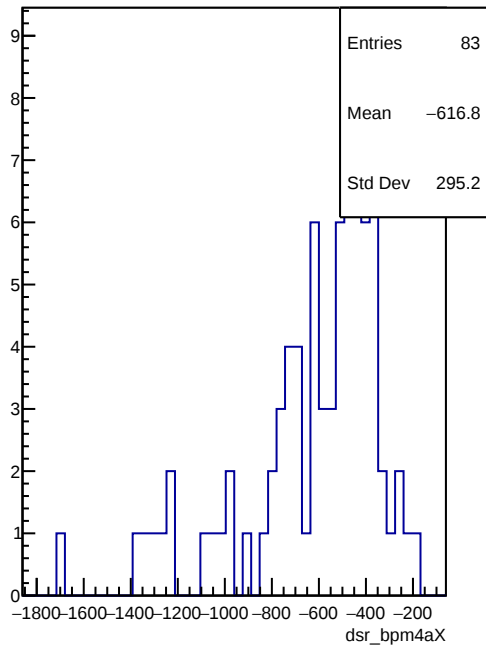
dsr_bpm4aX
