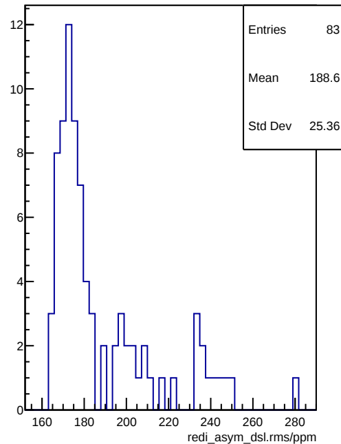
redi_asym_dsl.rms/ppm
