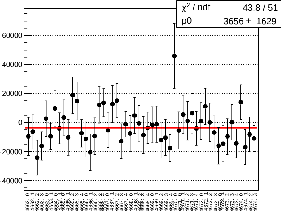
asym atl dd atr dd dd mean vs run
