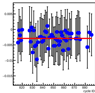
bpm4eX_coil6(um/count)
