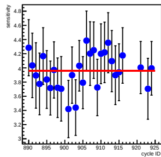
dsr_coil6(ppm/count)
