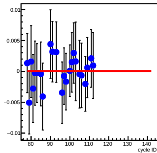
bpm8X_coil2(um/count)
