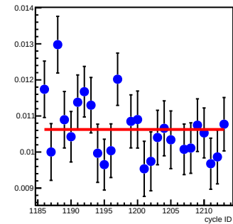
bpm16Y_coil7(um/count)
