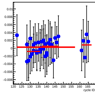
bpm8X_coil2(um/count)
