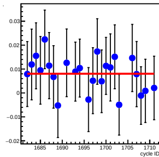
bpm4eX_coil6(um/count)
