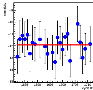
at1_coil6(ppm/count)
