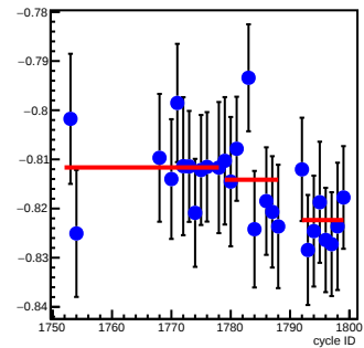
bpm12X_coil7(um/count)
