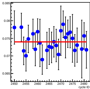
bpm1Y_coil7(um/count)
