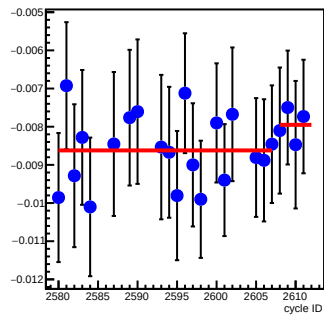
bpm16Y_coil7(um/count)
