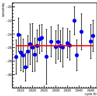
at1_coil6(ppm/count)
