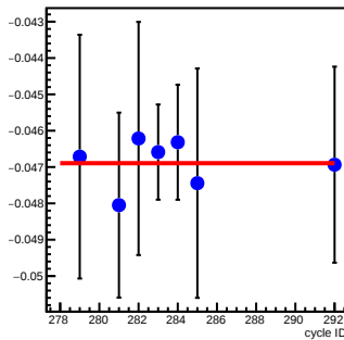
bpm1Y_coil5(um/count)
