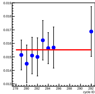
bpm4aY_coil7(um/count)
