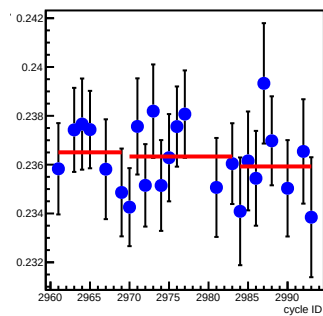
bpm11Y_coil6(um/count)
