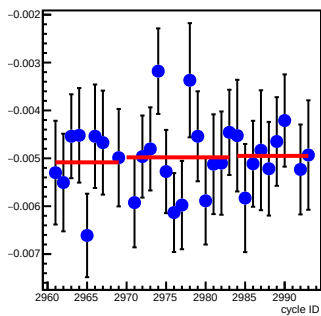
bpm11Y_coil2(um/count)
