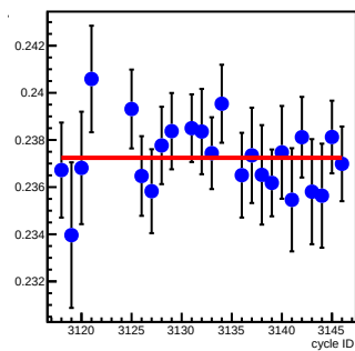
bpm11Y_coil6(um/count)
