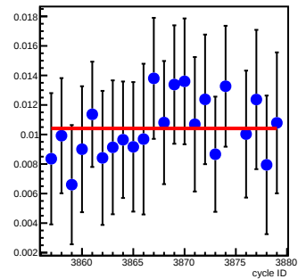
bpm4eY_coil5(um/count)
