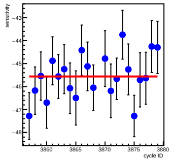
usl_coil7(ppm/count)
