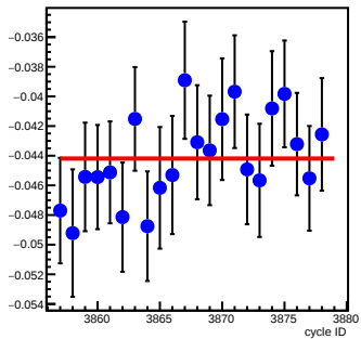
bpm4aX_coil7(um/count)
