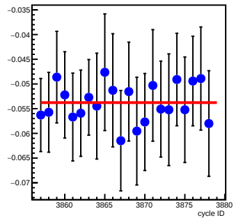
bpm12Y_coil7(um/count)
