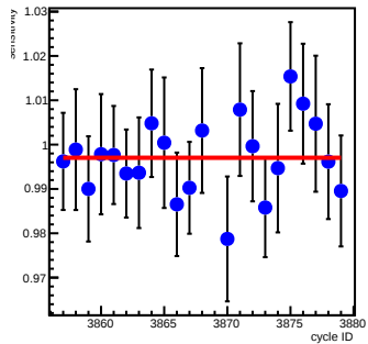
bpm4eX_coil7(um/count)
