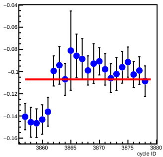
bpm1Y_coil7(um/count)
