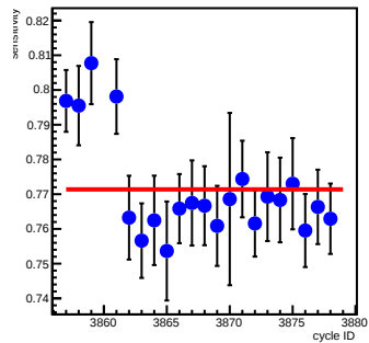
bpm1Y_coil6(um/count)
