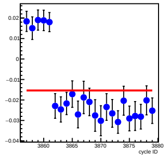
bpm1Y_coil2(um/count)
