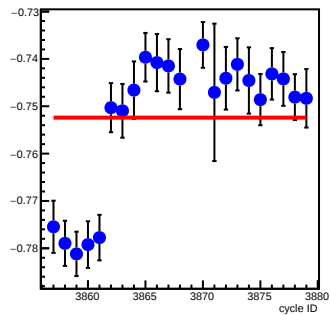
bpm1Y_coil2(um/count)
