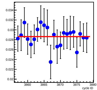
bpm16Y_coil7(um/count)
