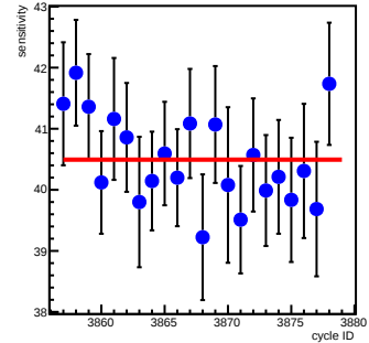
usr_coil7(ppm/count)
