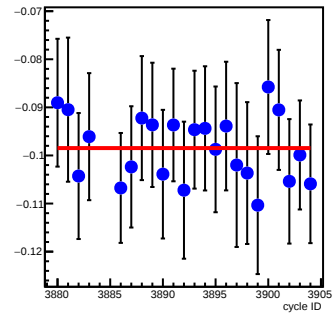
bpm1Y_coil7(um/count)
