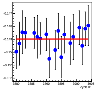
bpm11Y_coil5(um/count)
