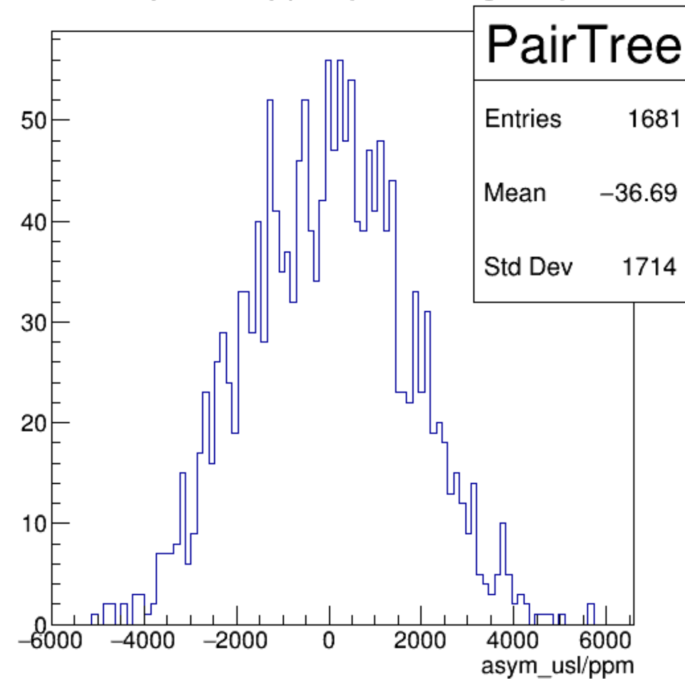
asym_usl/ppm {ErrorFlag==0}
