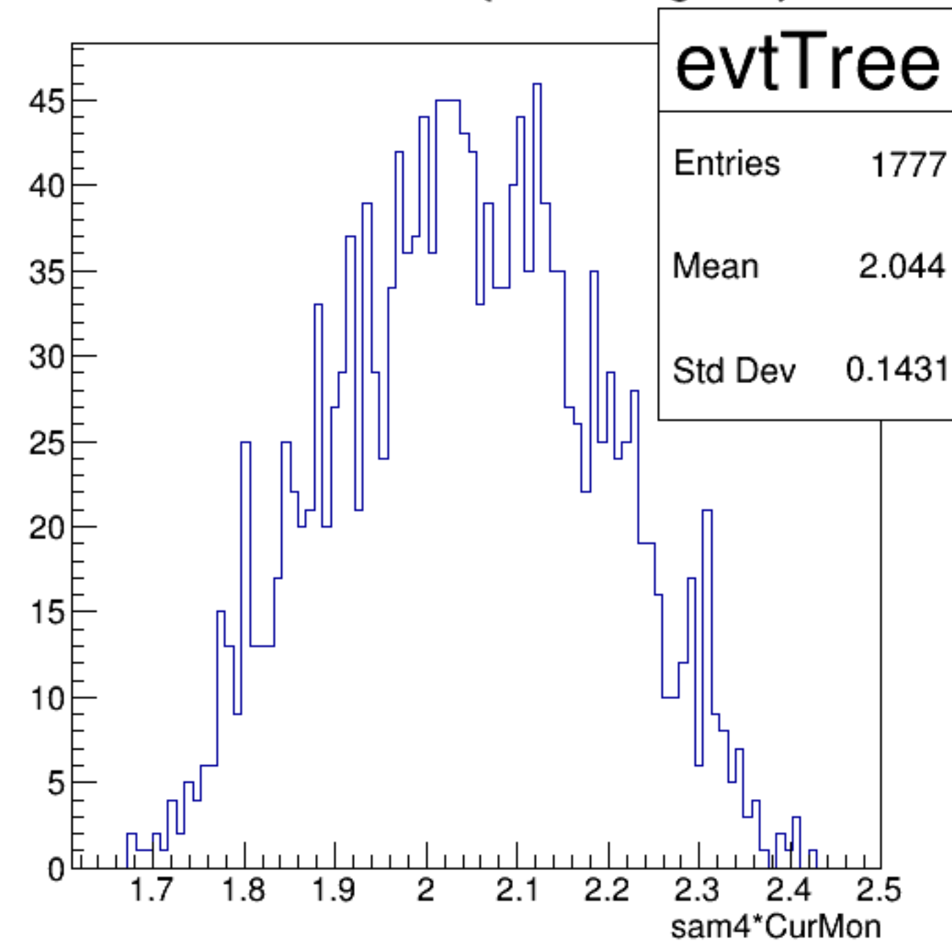
sam4*CurMon {ErrorFlag==0}
