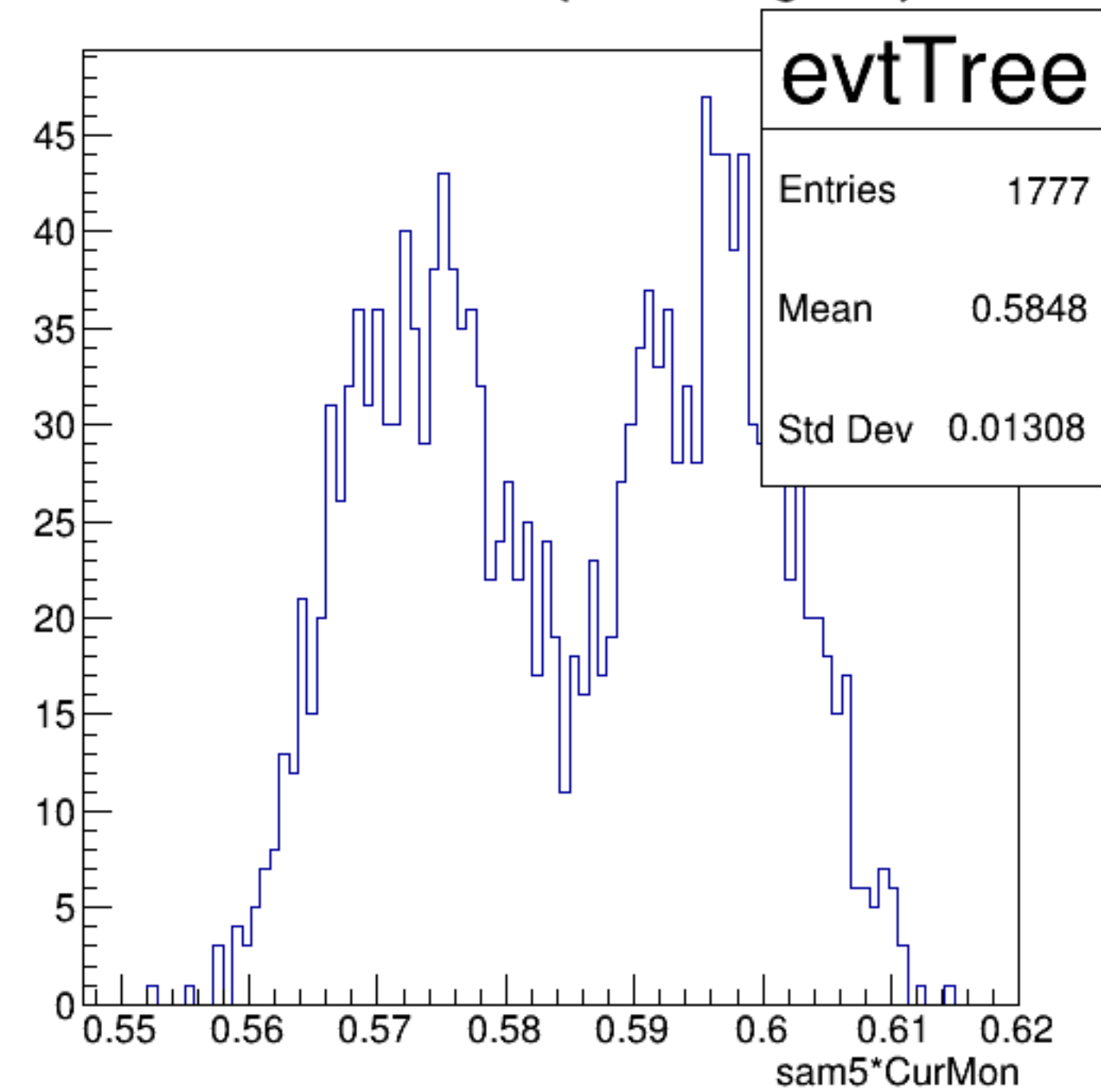
sam5*CurMon {ErrorFlag==0}
