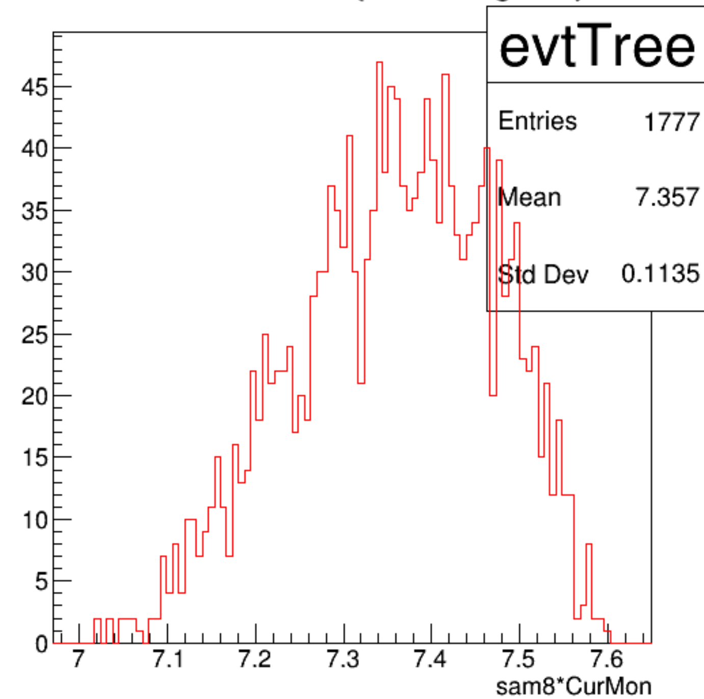
sam8*CurMon {ErrorFlag==0}
