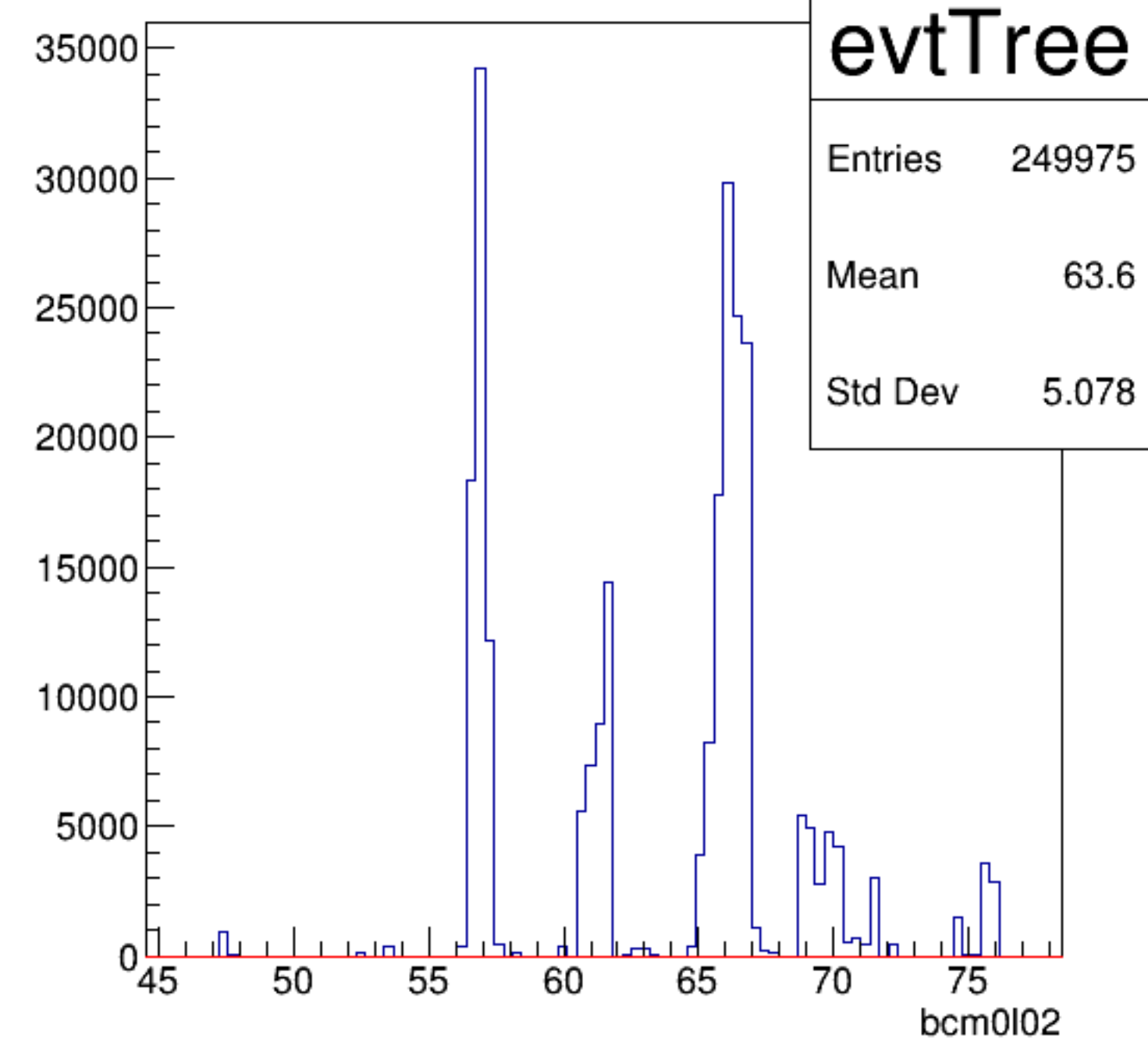
bcm0l02 {ErrorFlag==0}
