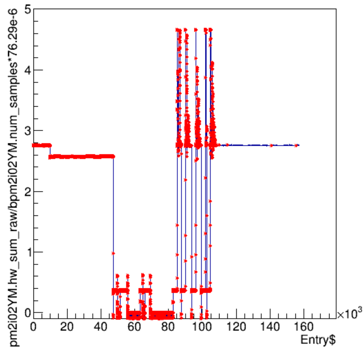
bpm2i02YM.hw_sum_raw/bpm2i02YM.num_samples*76.29e-6:Entry$
