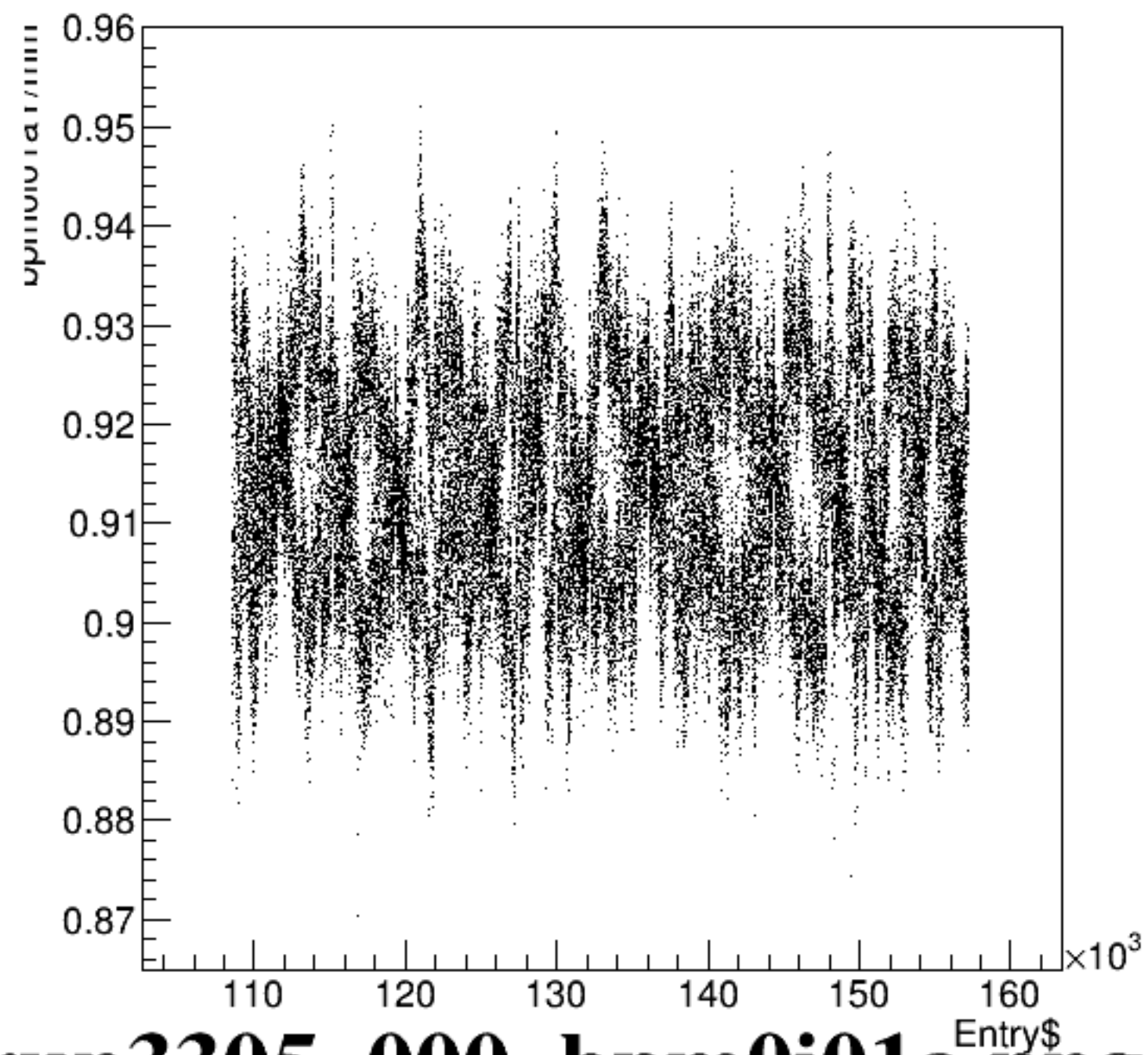
bpm0i01aY/mm:Entry$ {ErrorFlag==0}
