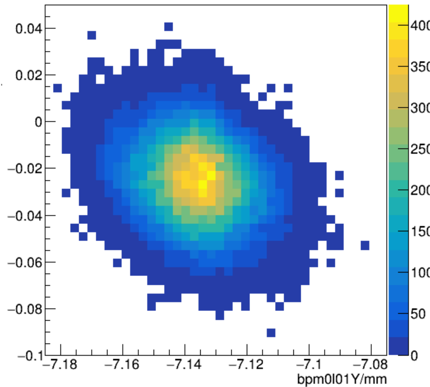
bpm0l01X/mm:bpm0l01Y/mm {ErrorFlag==0}
