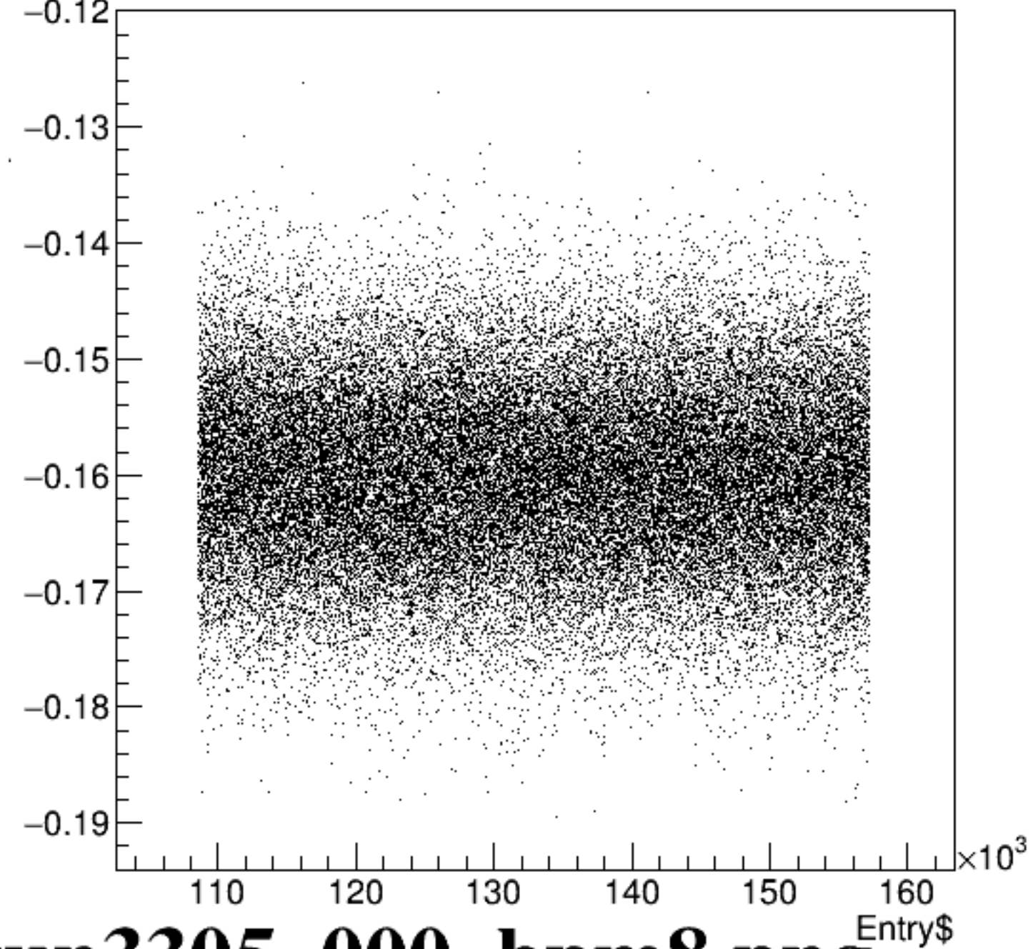
bpm8Y/mm:Entry$ {ErrorFlag==0}
