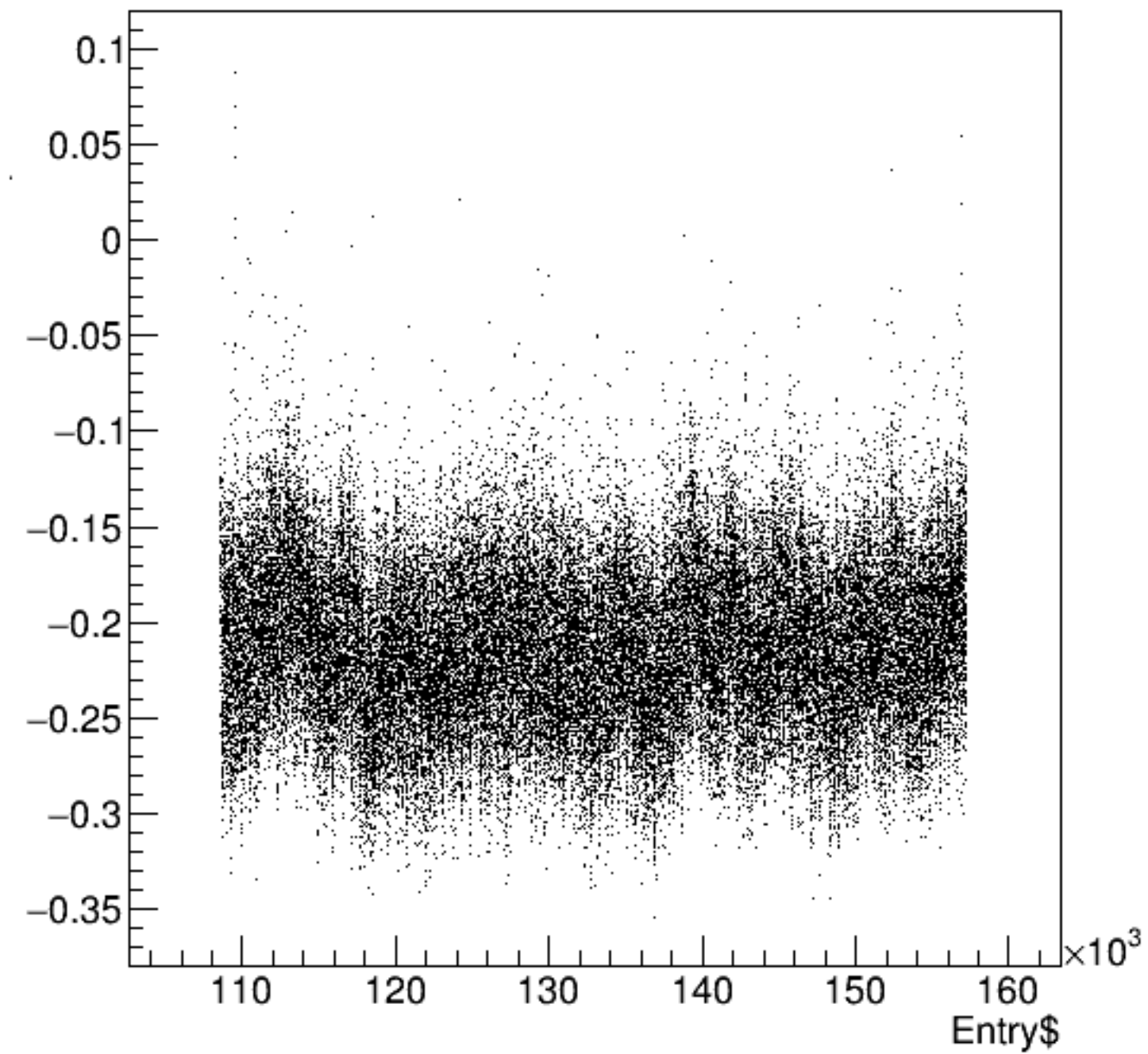
bpm8X/mm:Entry$ {ErrorFlag==0}
