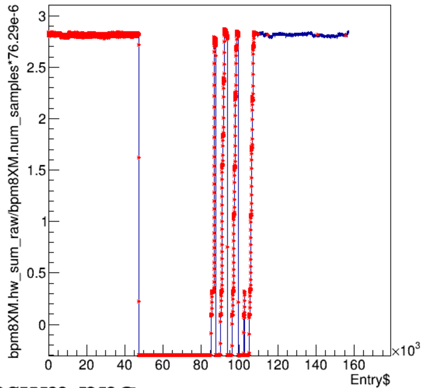
bpm8XM.hw_sum_raw/bpm8XM.num_samples*76.29e-6:Entry$
