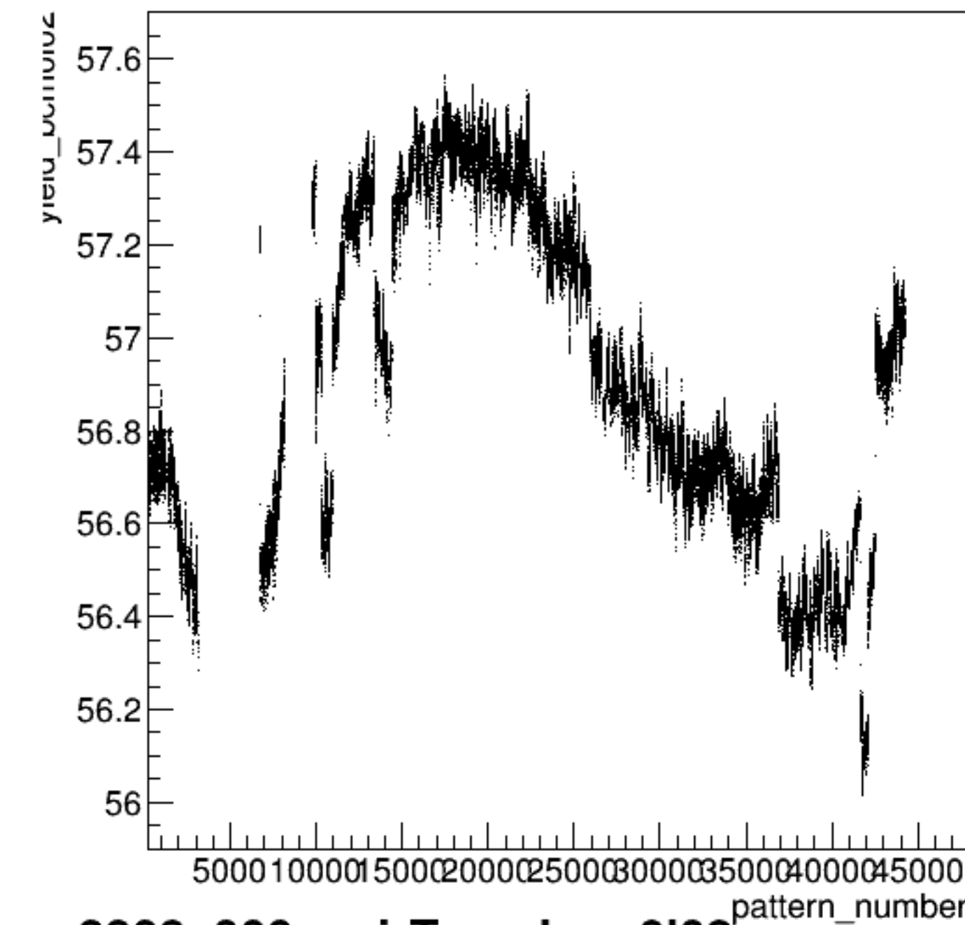
run3308_000_pairTree_bcm0l02.png
