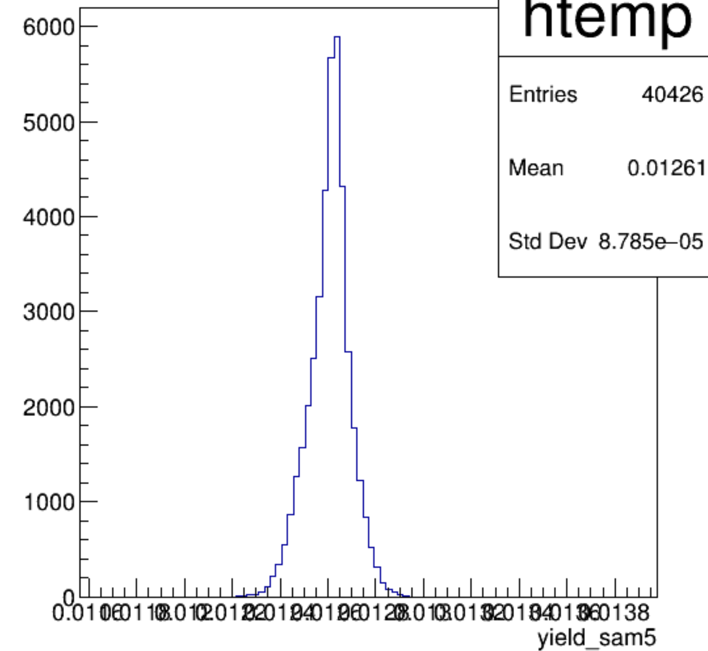
yield_sam5 {ErrorFlag==0}
