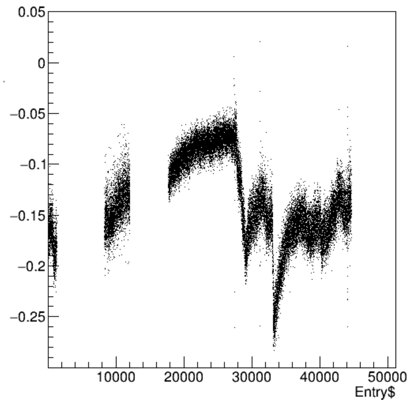
bpm14X/mm:Entry$ {ErrorFlag==0}
