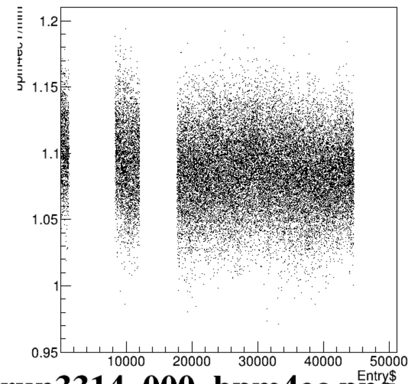
bpm4ecY/mm:Entry$ {ErrorFlag==0}
