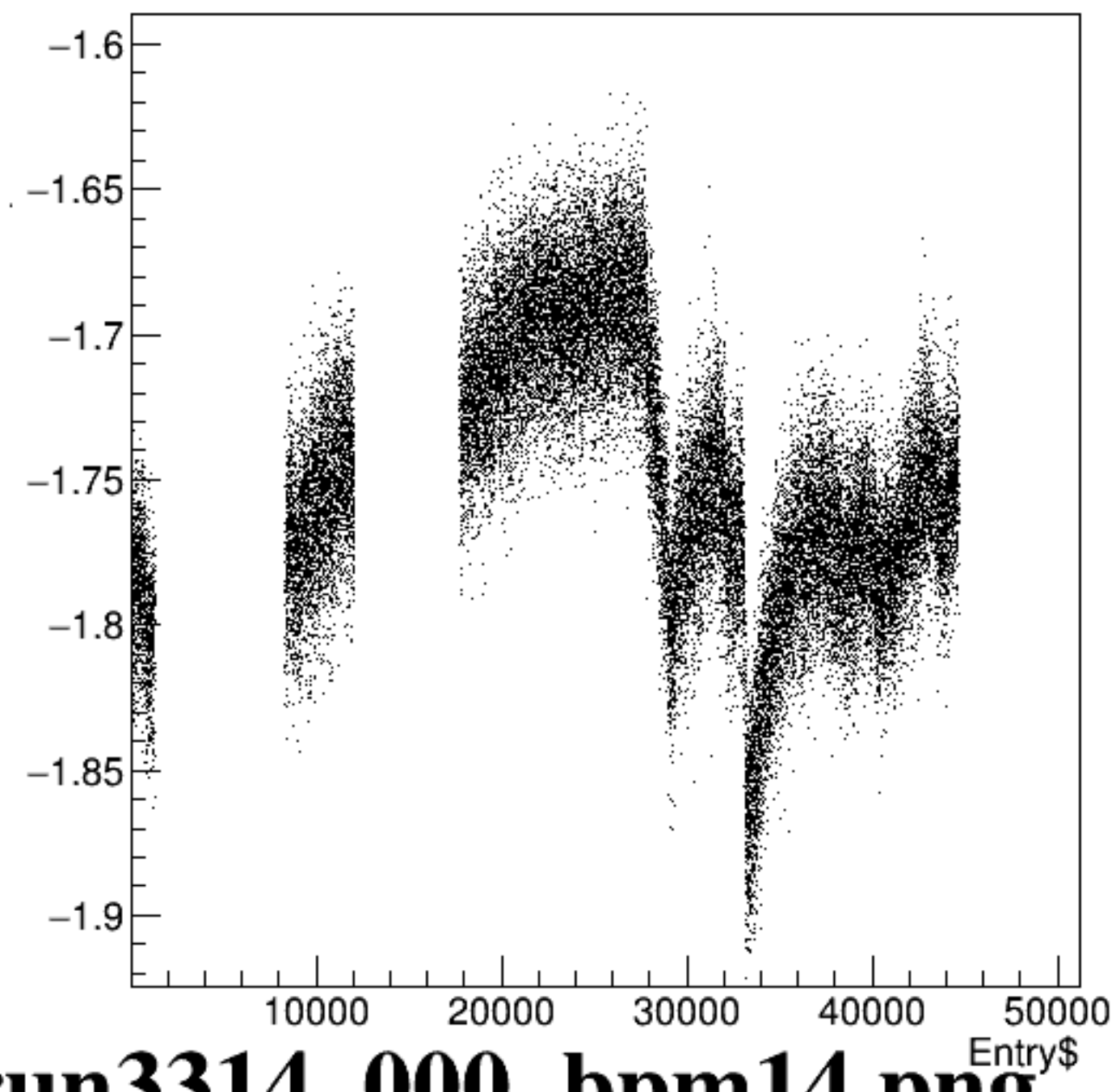
bpm14Y/mm:Entry$ {ErrorFlag==0}
