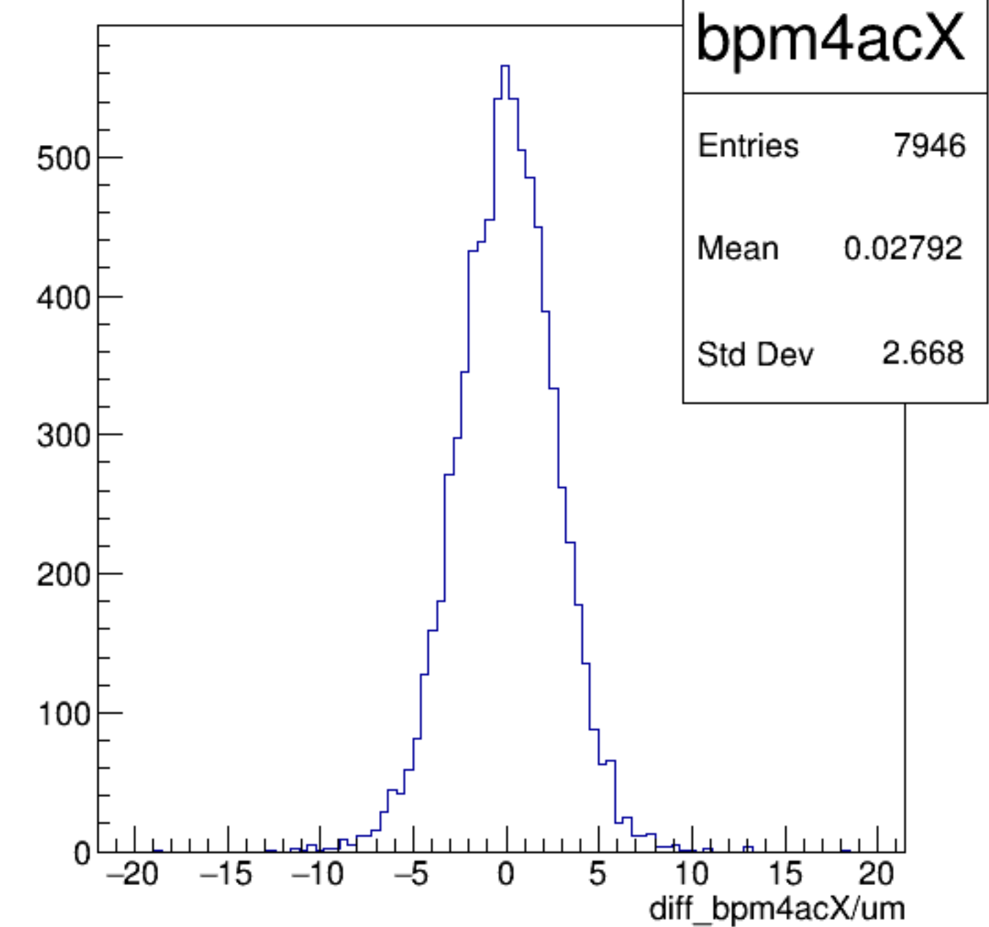
diff_bpm4acX/um {ErrorFlag==0}
