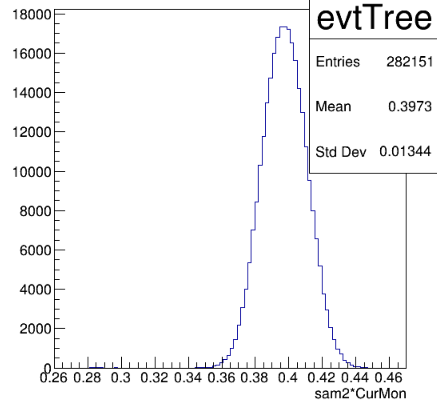
sam2*CurMon {ErrorFlag==0}
