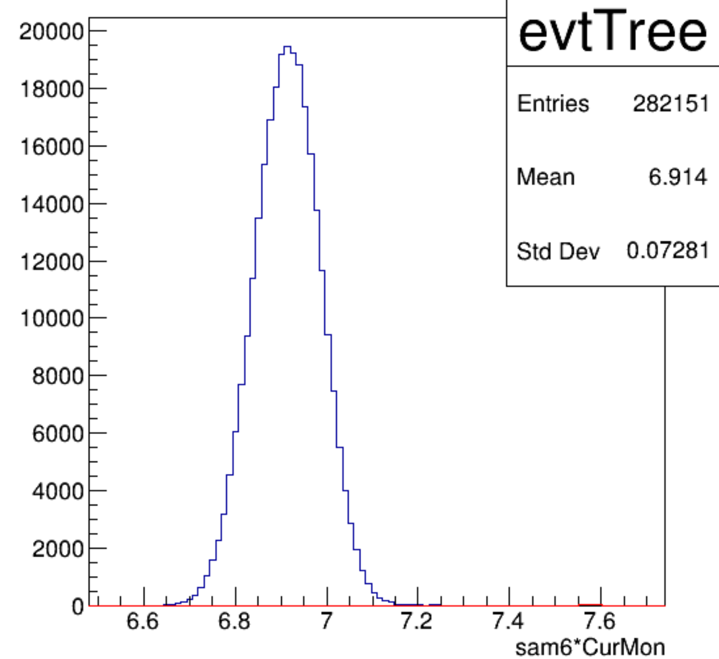
sam6*CurMon {ErrorFlag==0}
