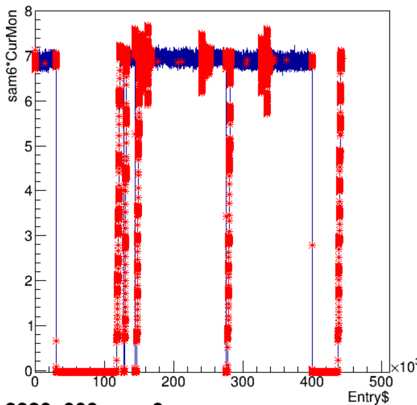
sam6*CurMon:Entry$
