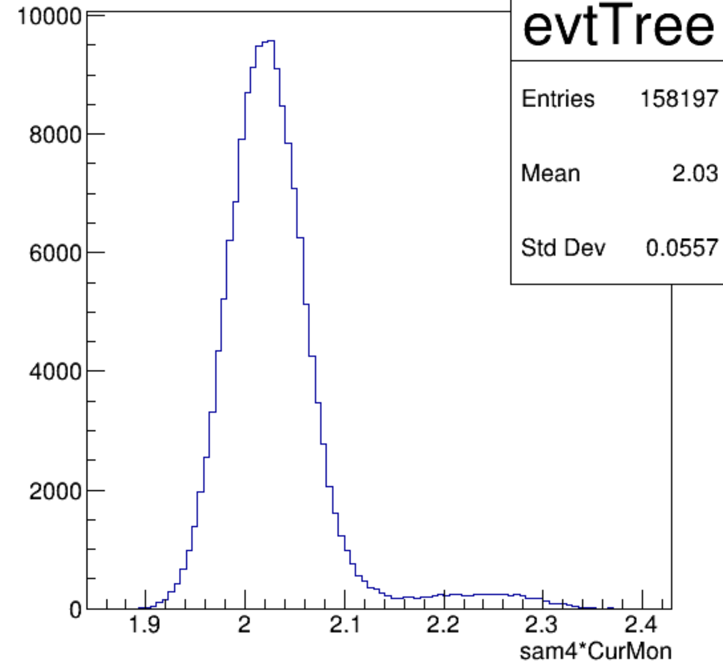
sam4*CurMon {ErrorFlag==0}
