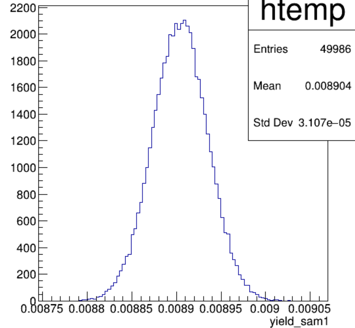
yield_sam1 {ErrorFlag==0}
