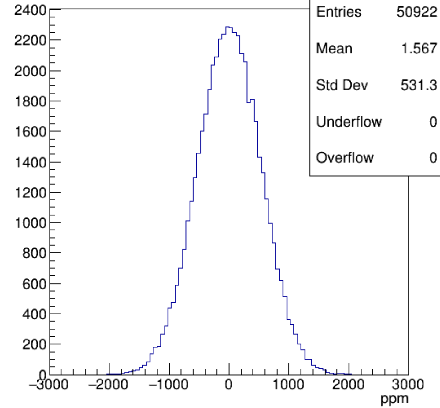
asym_usl
