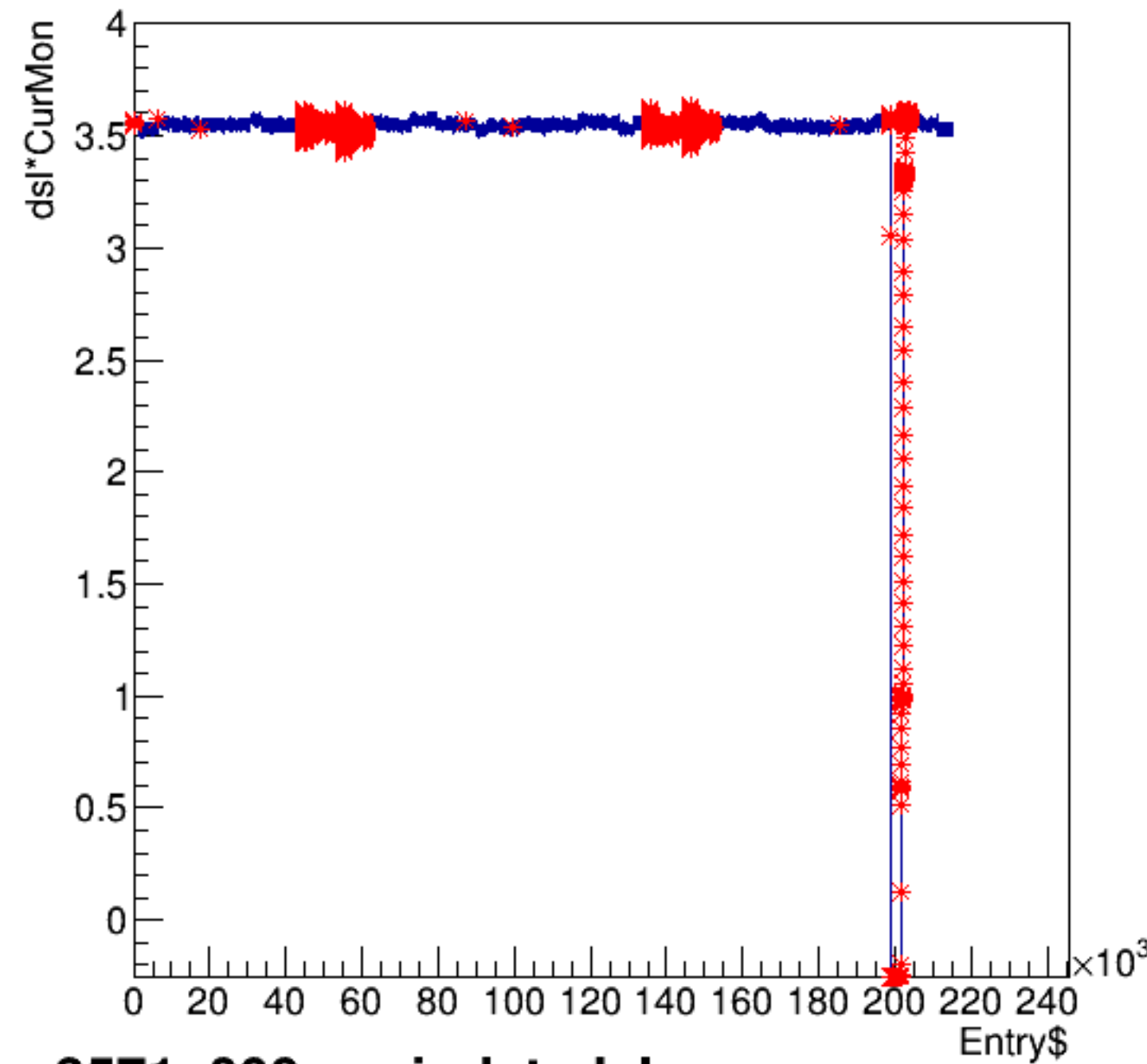
dsl*CurMon:Entry$
