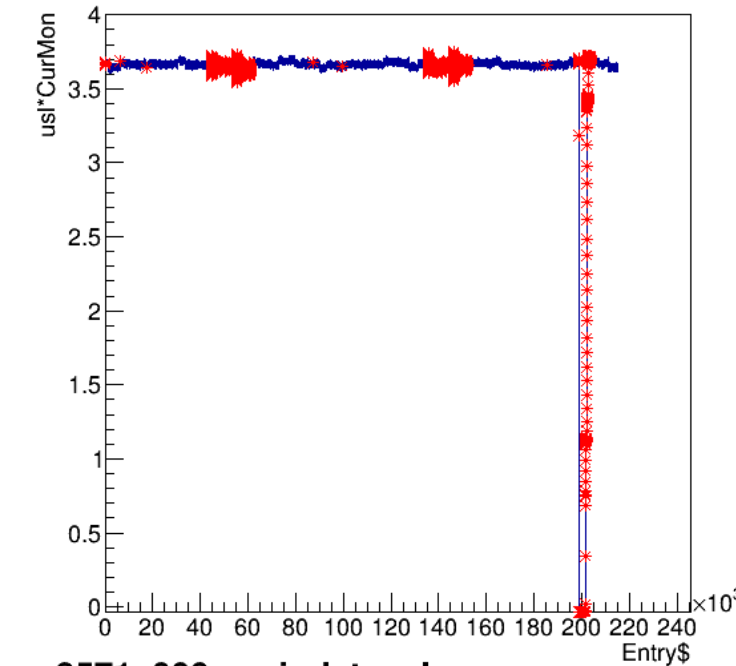
usl*CurMon:Entry$
