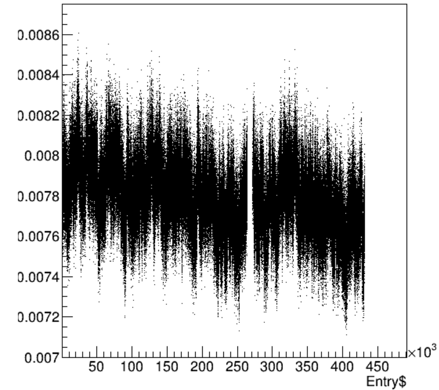
bpm4acX/mm:Entry$ {ErrorFlag==0}
