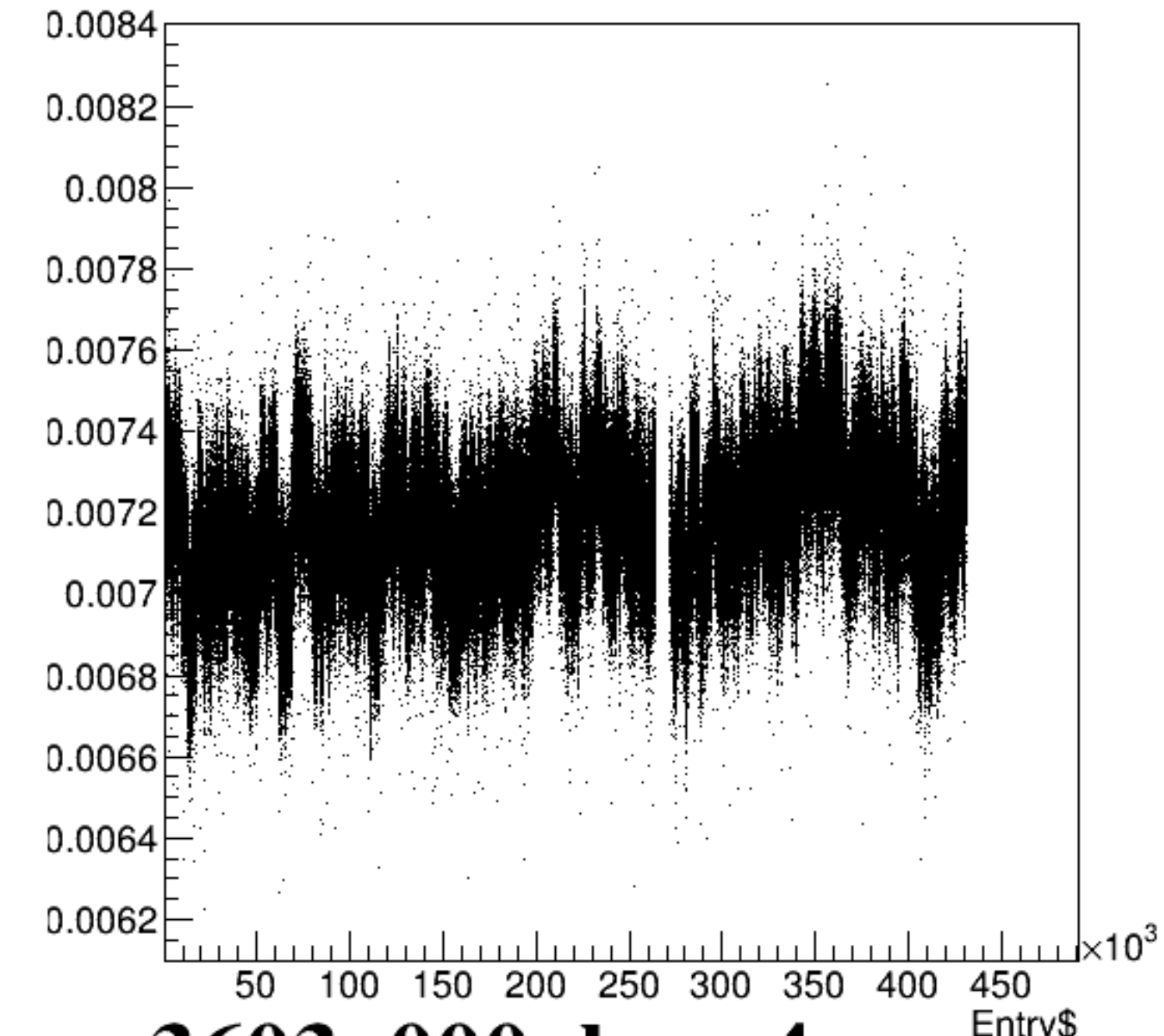
bpm4acY/mm:Entry$ {ErrorFlag==0}
