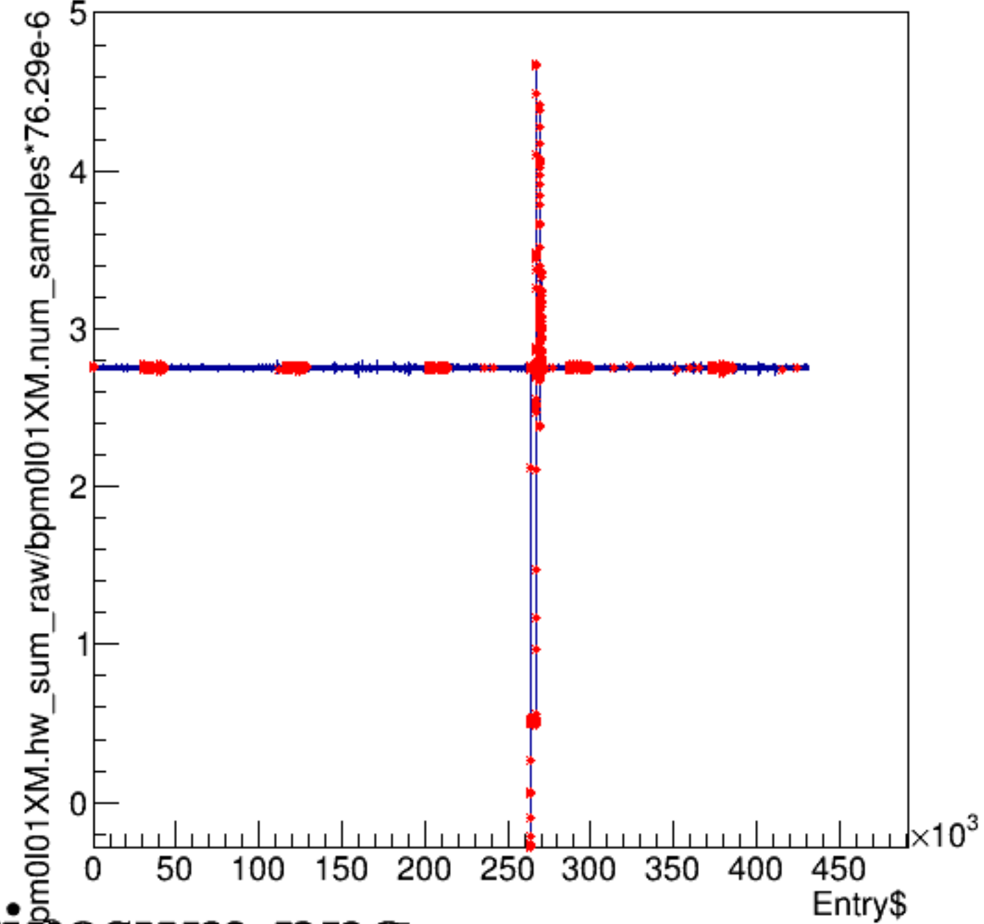
bpm0l01XM.hw_sum_raw/bpm0l01XM.num_samples*76.29e-6:Entry$
