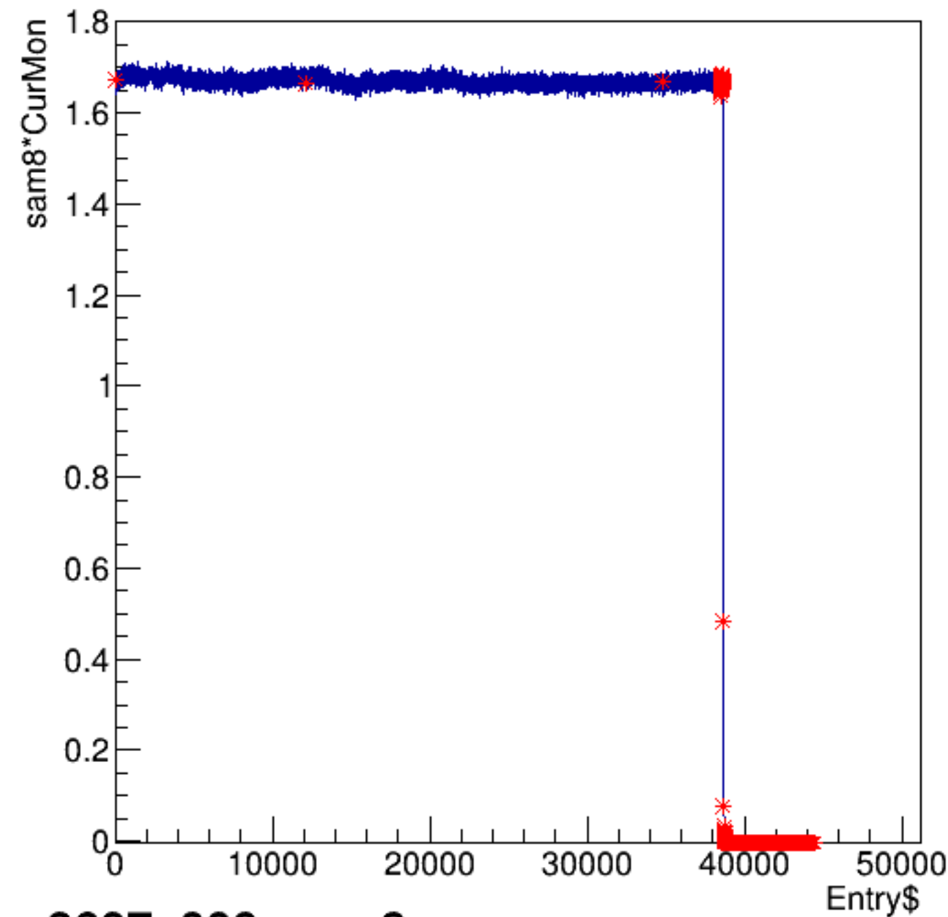
sam8*CurMon:Entry$
