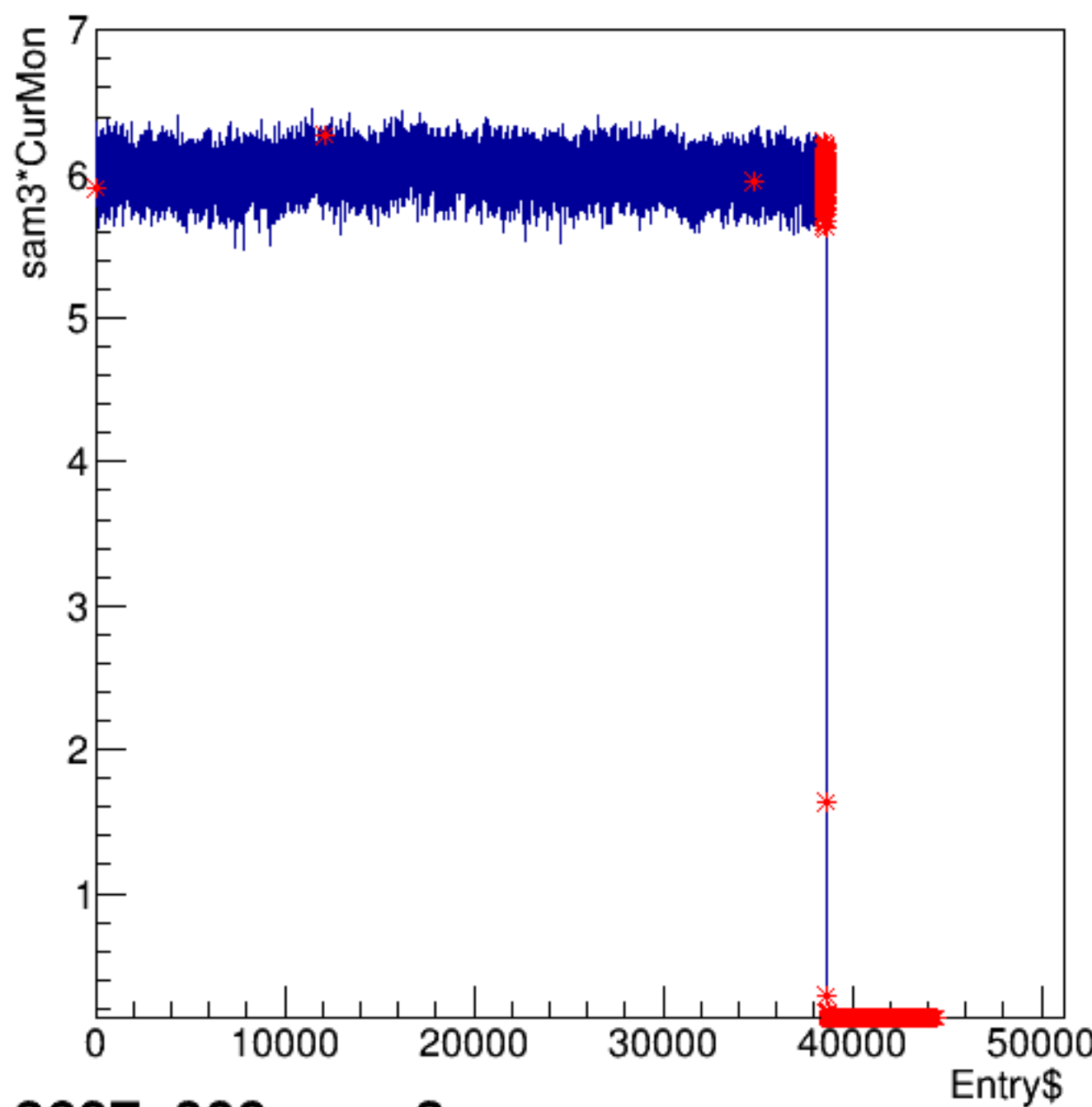
sam3*CurMon:Entry$
