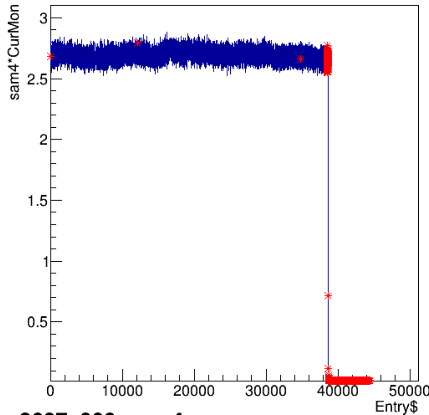
sam4*CurMon:Entry$
