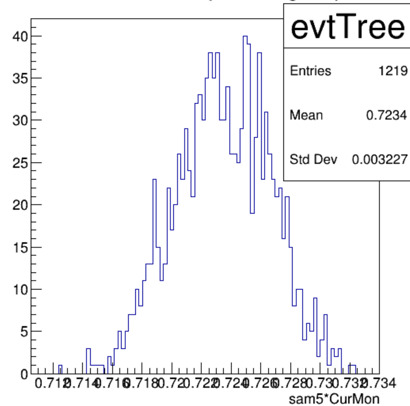
sam5*CurMon {ErrorFlag==0}
