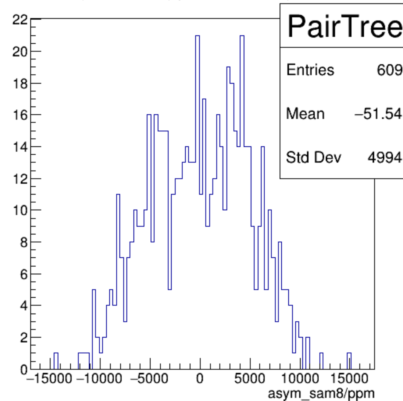
asym_sam8/ppm {ErrorFlag==0}
