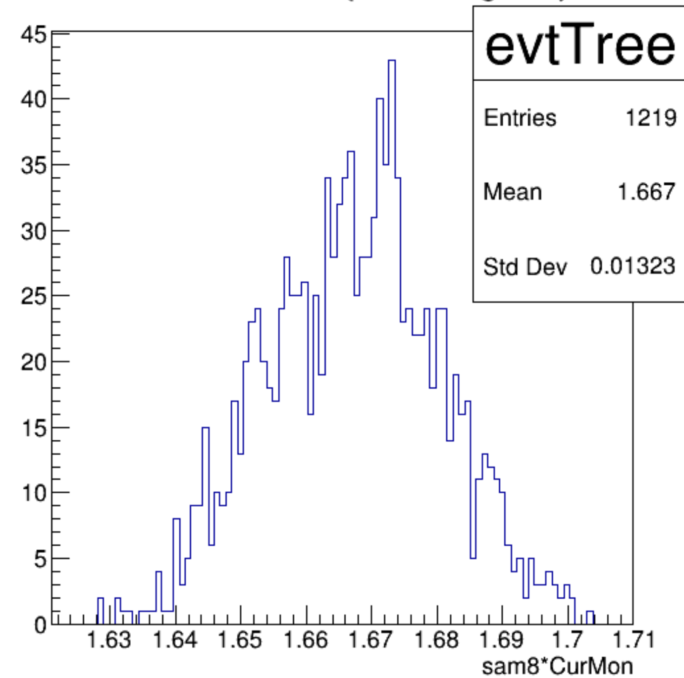
sam8*CurMon {ErrorFlag==0}
