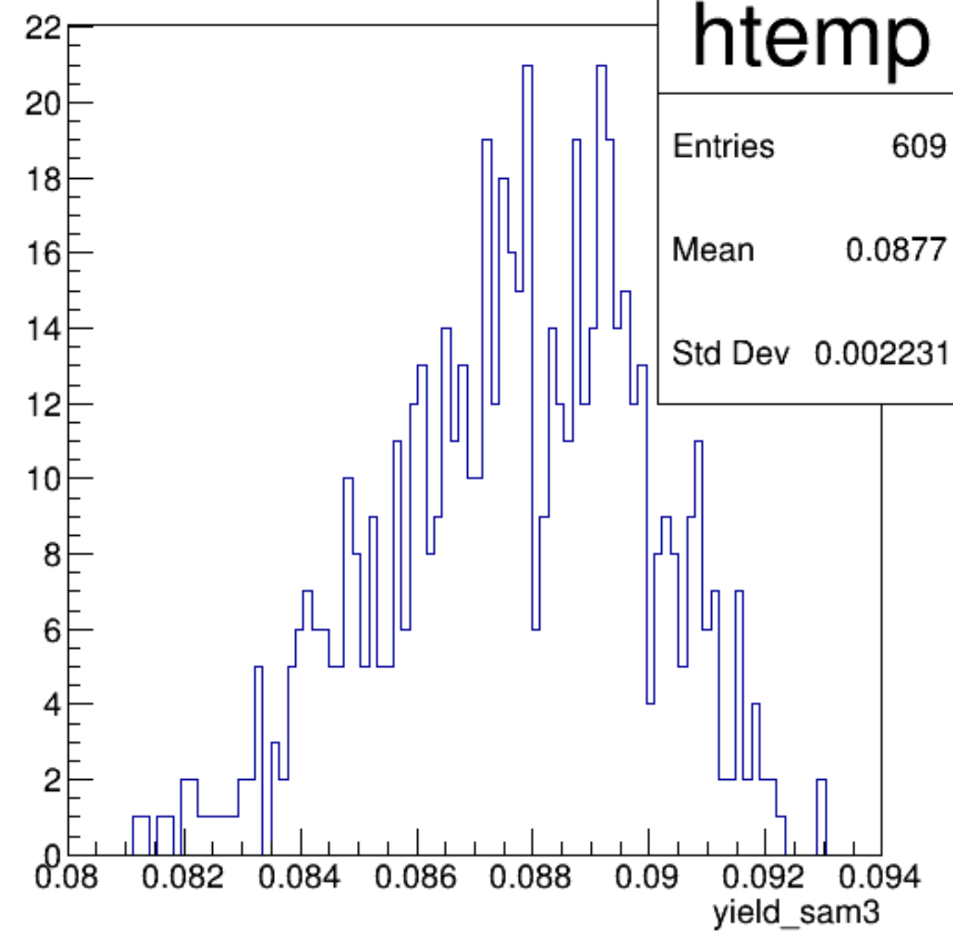
yield_sam3 {ErrorFlag==0}
