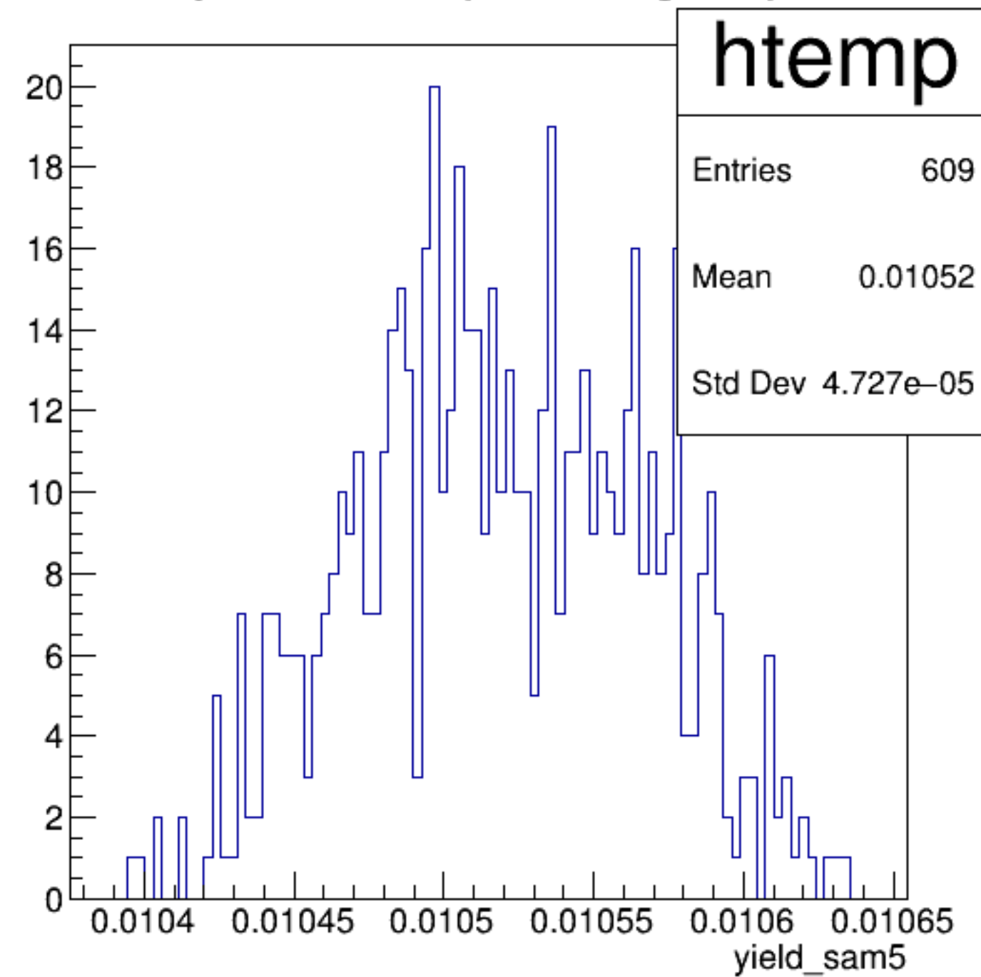
yield_sam5 {ErrorFlag==0}
