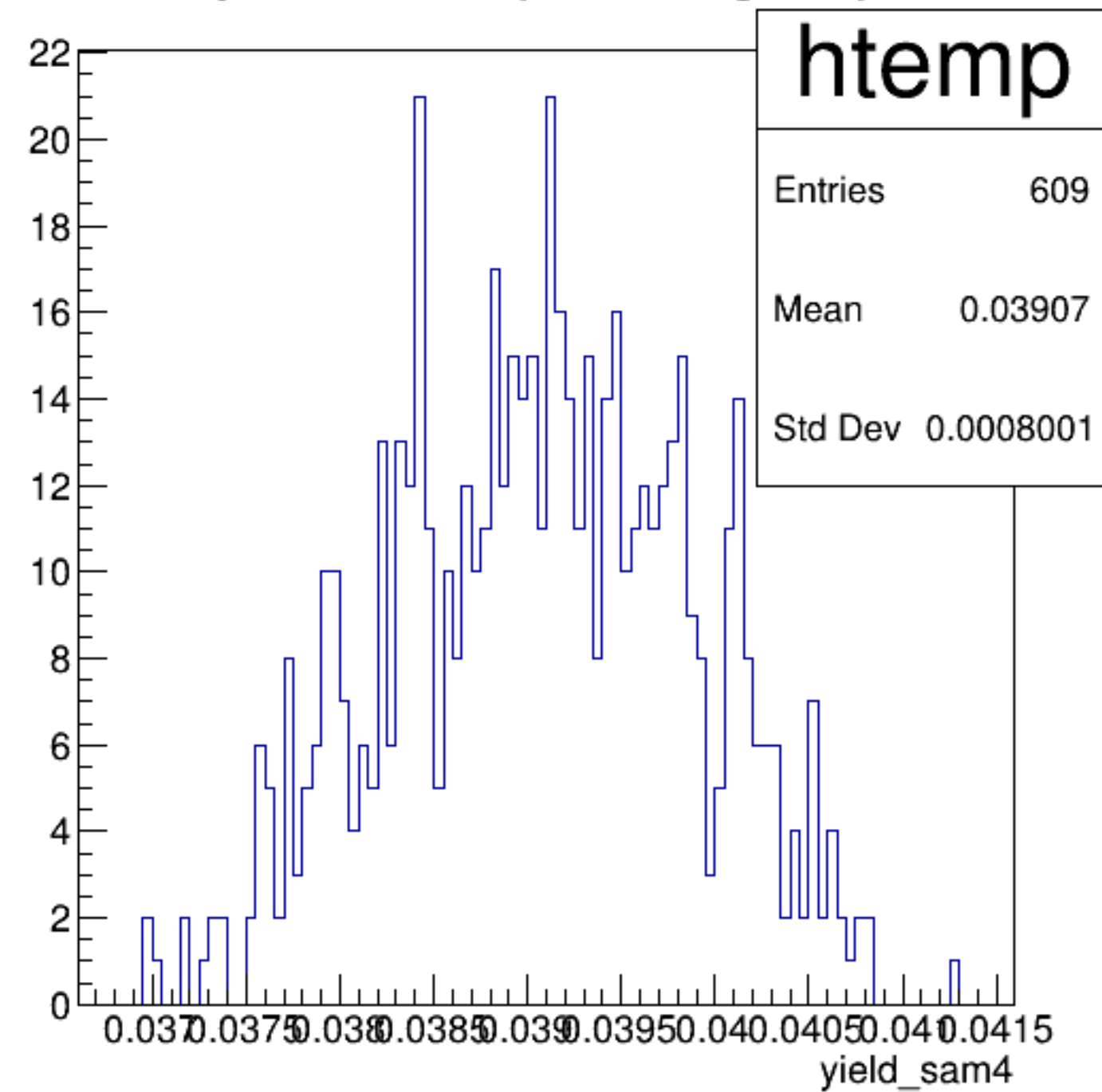
yield_sam4 {ErrorFlag==0}
