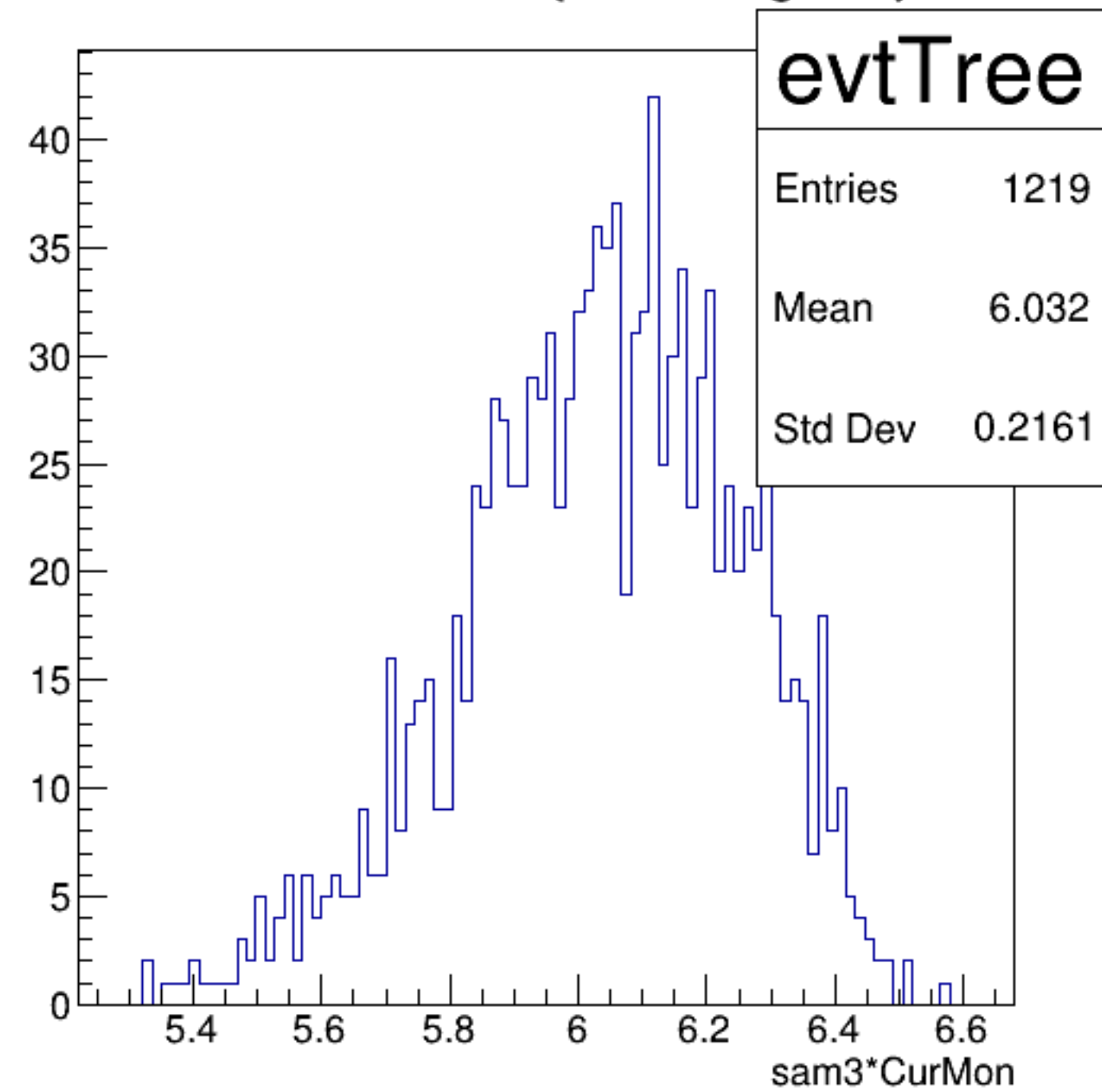
sam3*CurMon {ErrorFlag==0}
