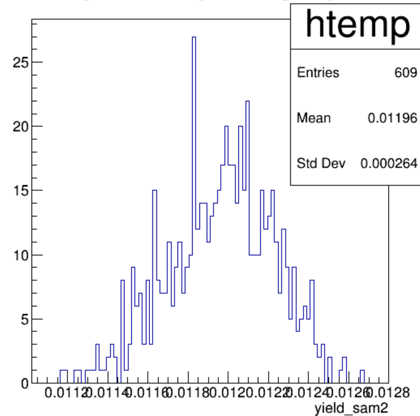
yield_sam2 {ErrorFlag==0}
