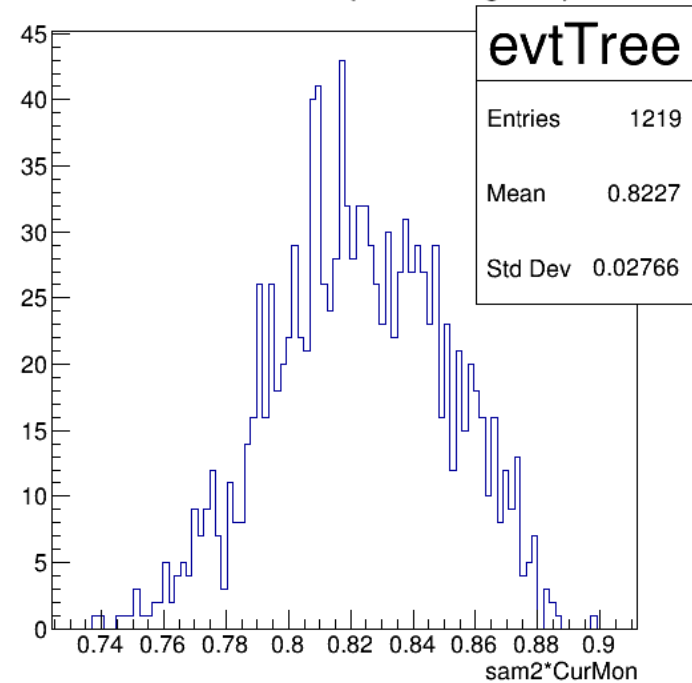
sam2*CurMon {ErrorFlag==0}
