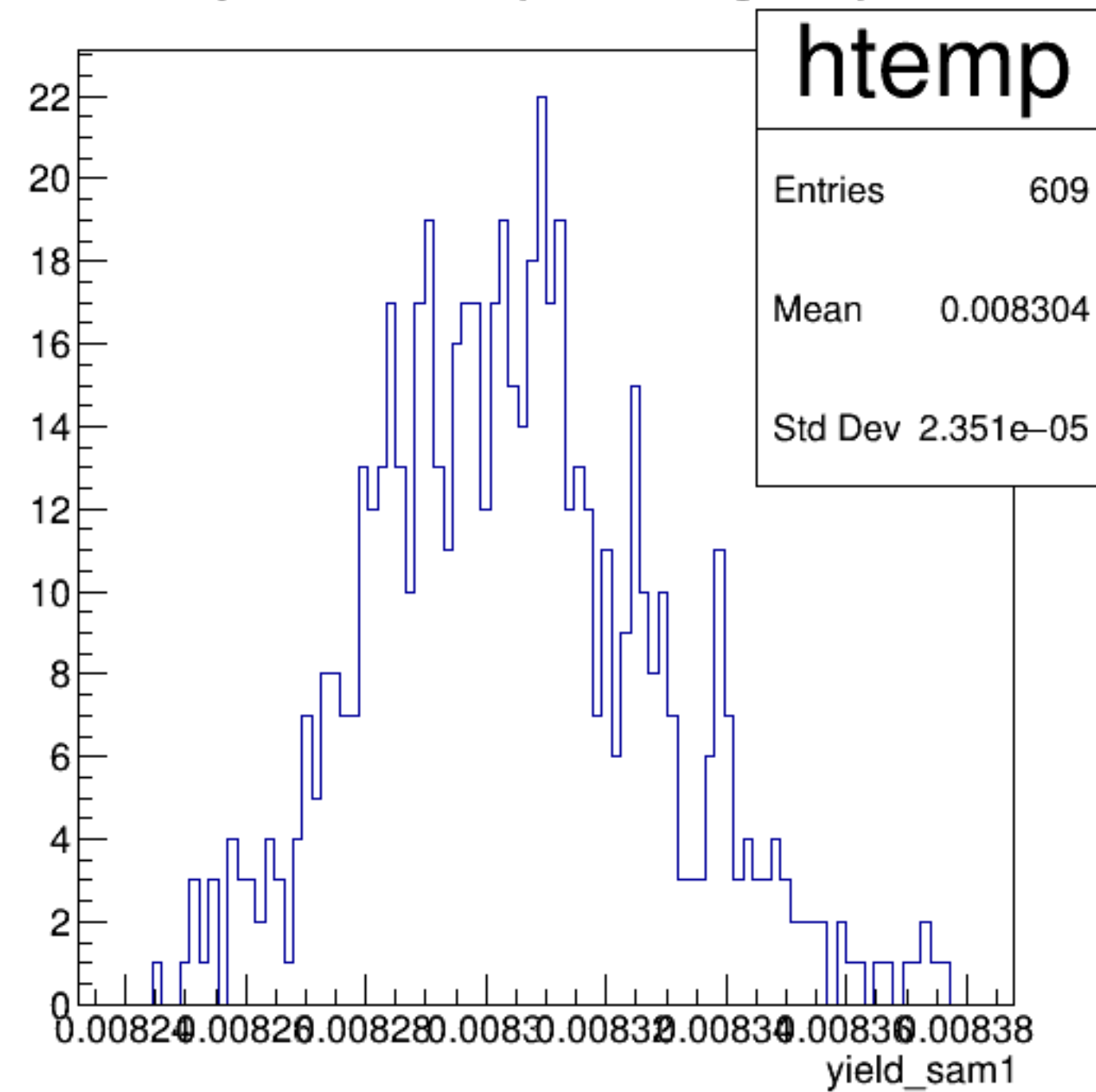
yield_sam1 {ErrorFlag==0}
