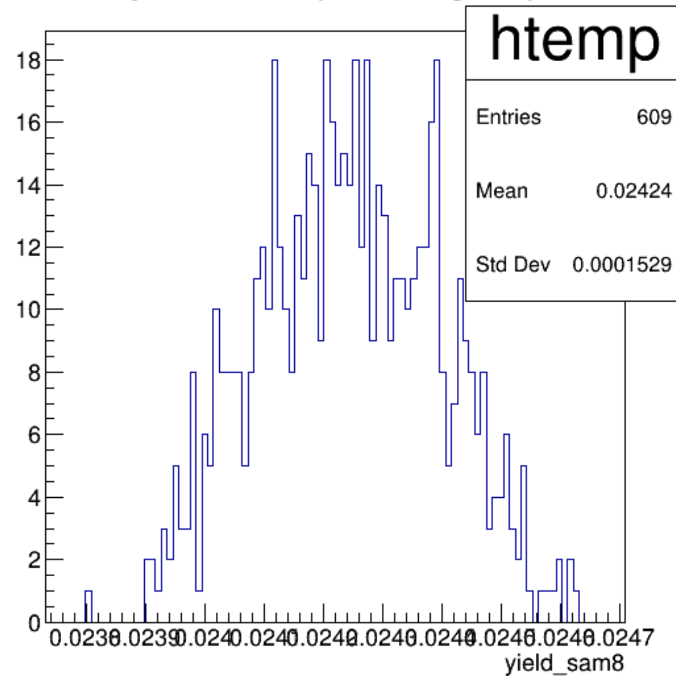
yield_sam8 {ErrorFlag==0}
