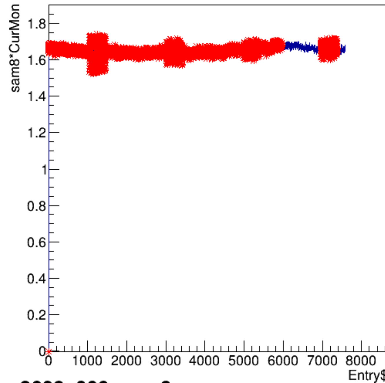
sam8*CurMon:Entry$
