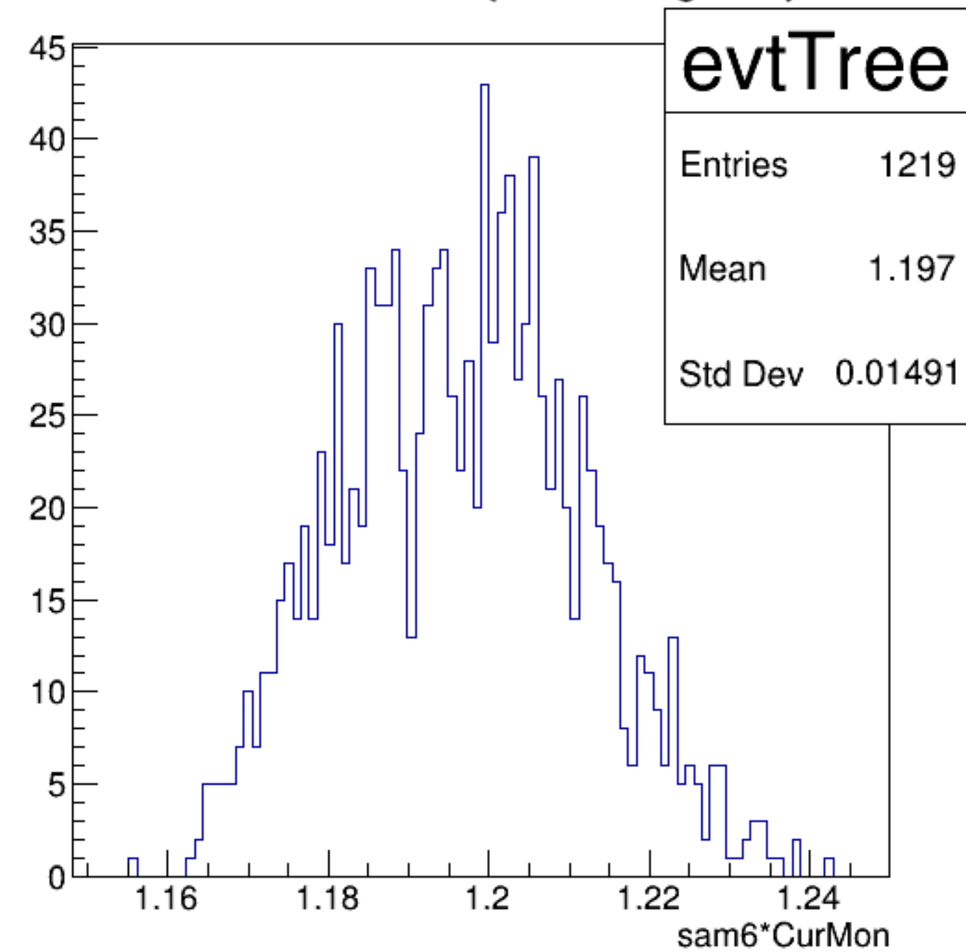
sam6*CurMon {ErrorFlag==0}
