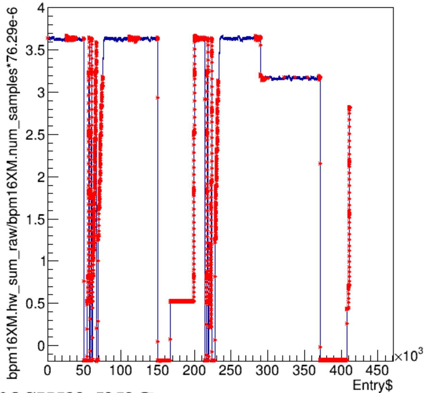
bpm16XM.hw_sum_raw/bpm16XM.num_samples*76.29e-6:Entry$
