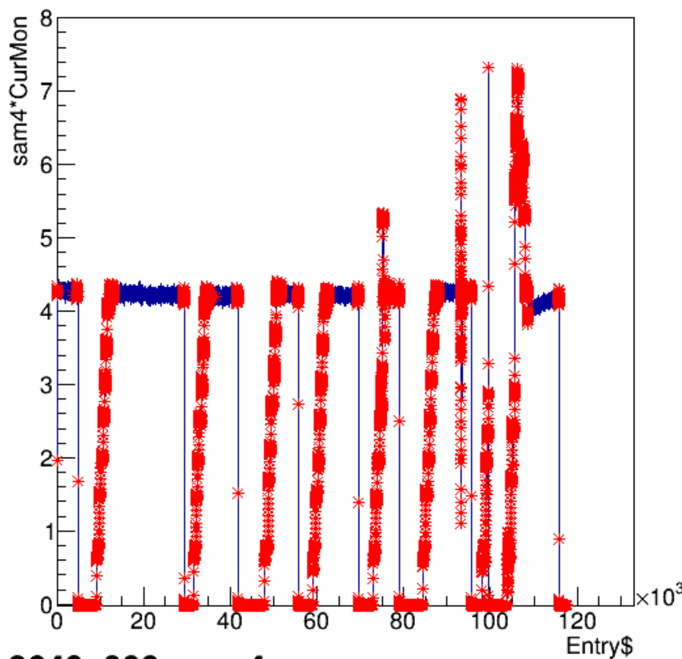
sam4*CurMon:Entry$
