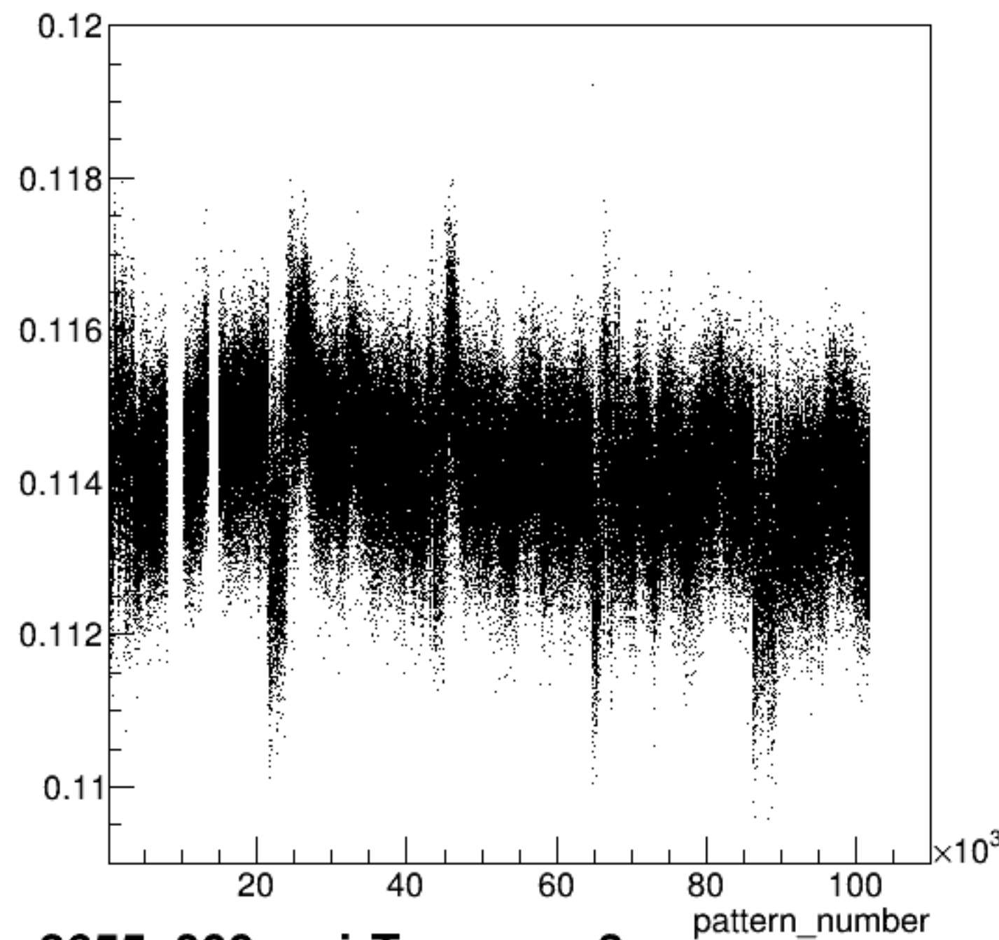
yield_sam3:pattern_number {ErrorFlag==0}
