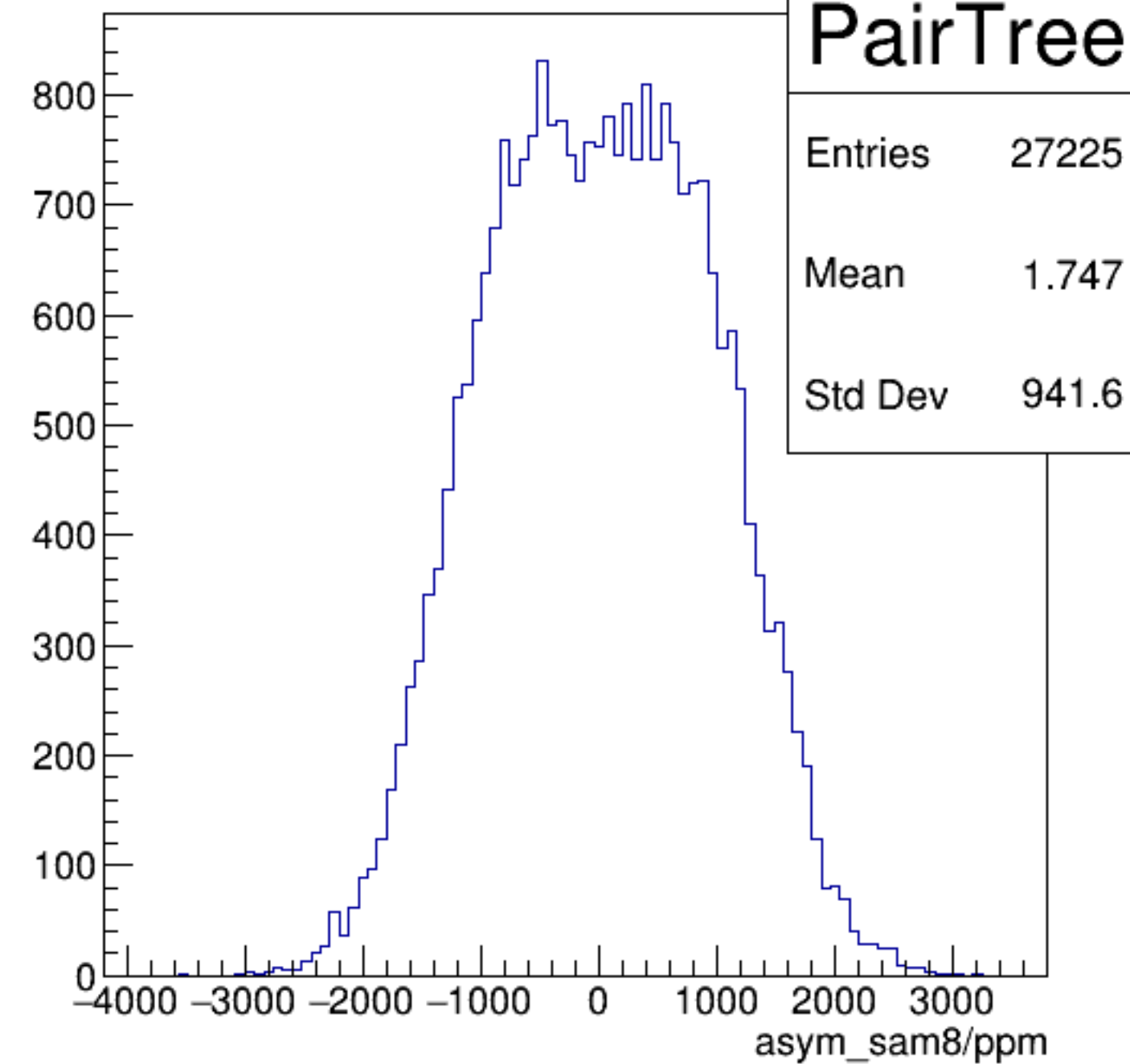
asym_sam8/ppm {ErrorFlag==0}
