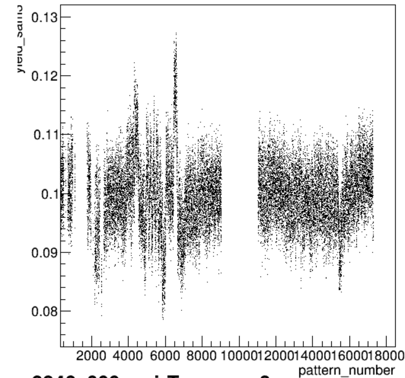
yield_sam3:pattern_number {ErrorFlag==0}
