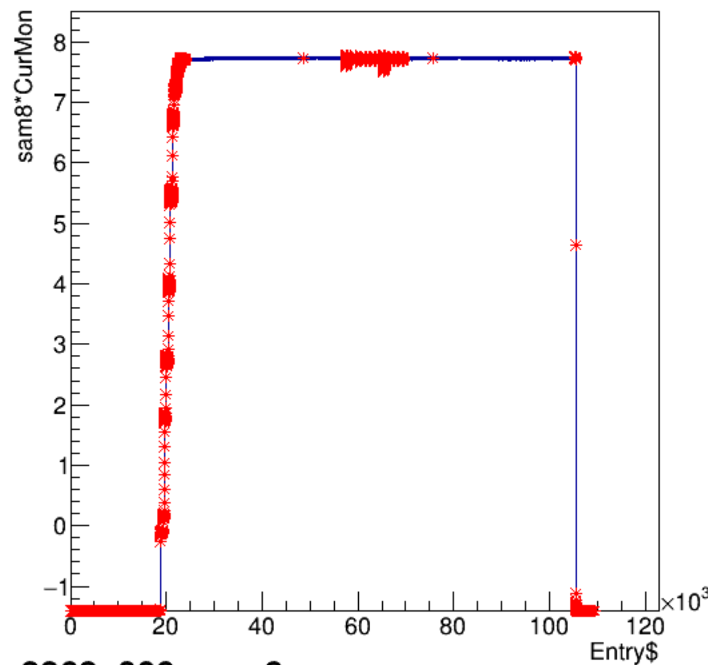
sam8*CurMon:Entry$
