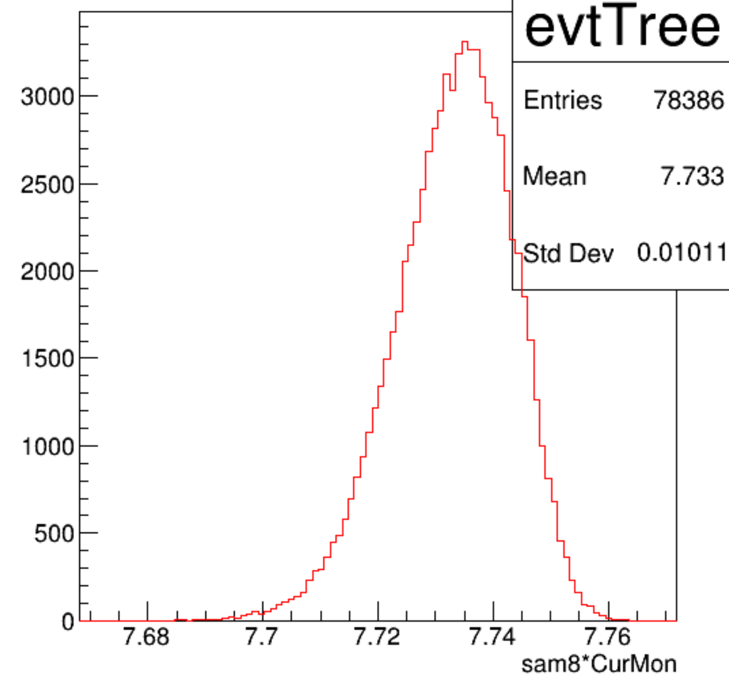
sam8*CurMon {ErrorFlag==0}
