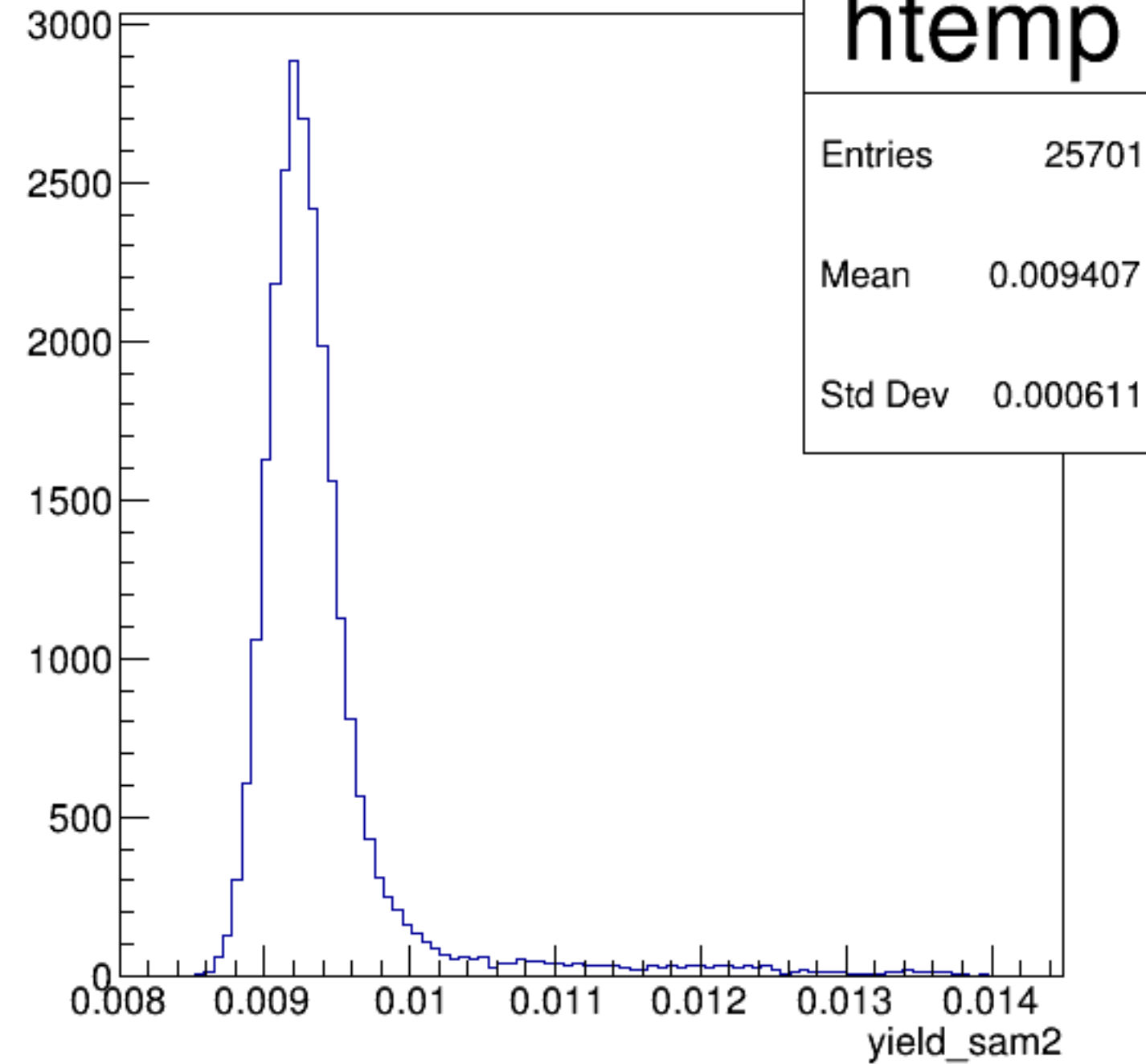
yield_sam2 {ErrorFlag==0}
