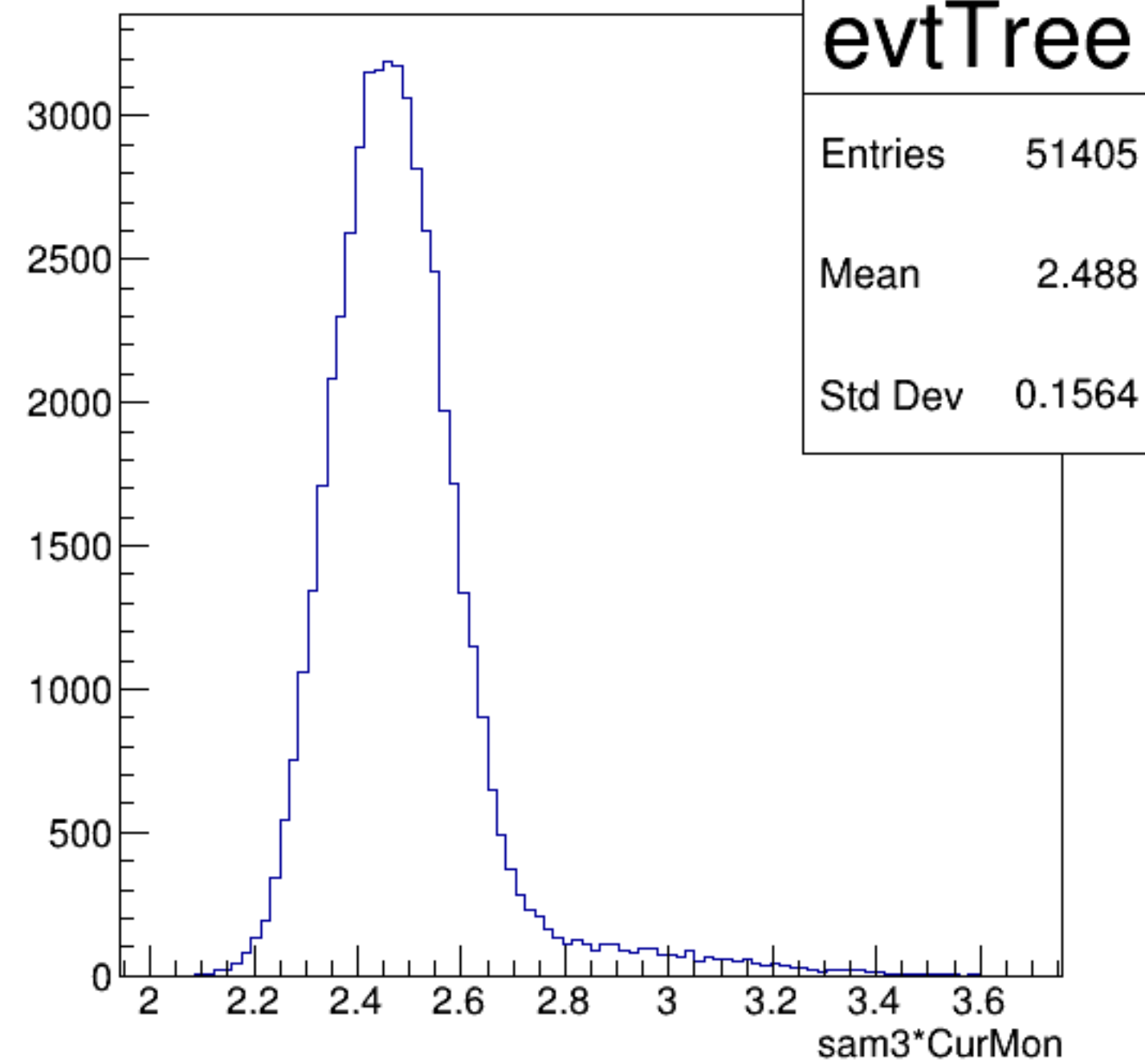
sam3*CurMon {ErrorFlag==0}
