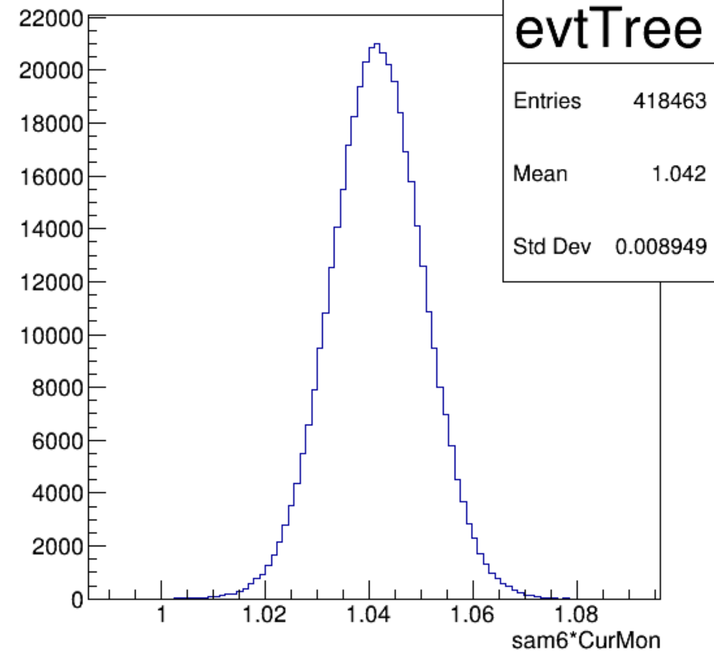
sam6*CurMon {ErrorFlag==0}
