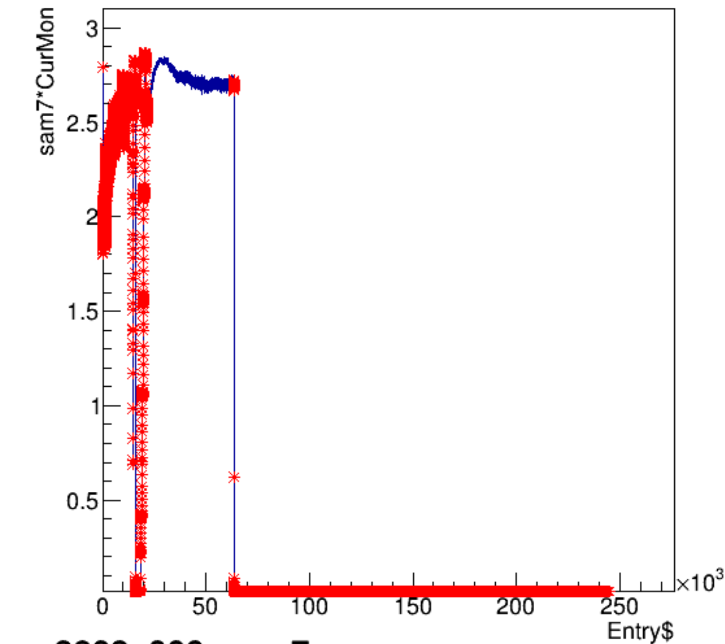
sam7*CurMon:Entry$
