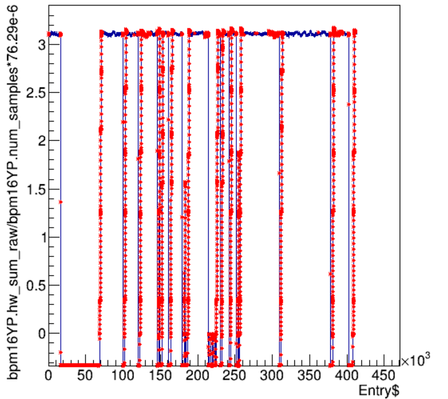
bpm16YP.hw_sum_raw/bpm16YP.num_samples*76.29e-6:Entry$
