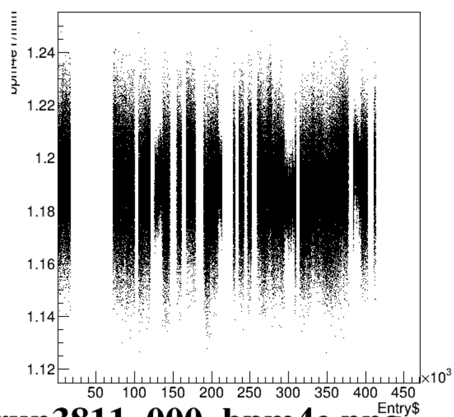
bpm4eY/mm:Entry$ {ErrorFlag==0}
