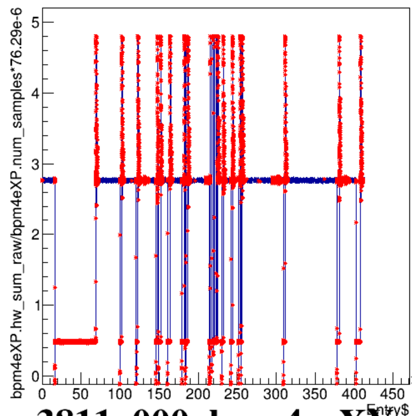
bpm4eXP.hw_sum_raw/bpm4eXP.num_samples*76.29e-6:Entry$
