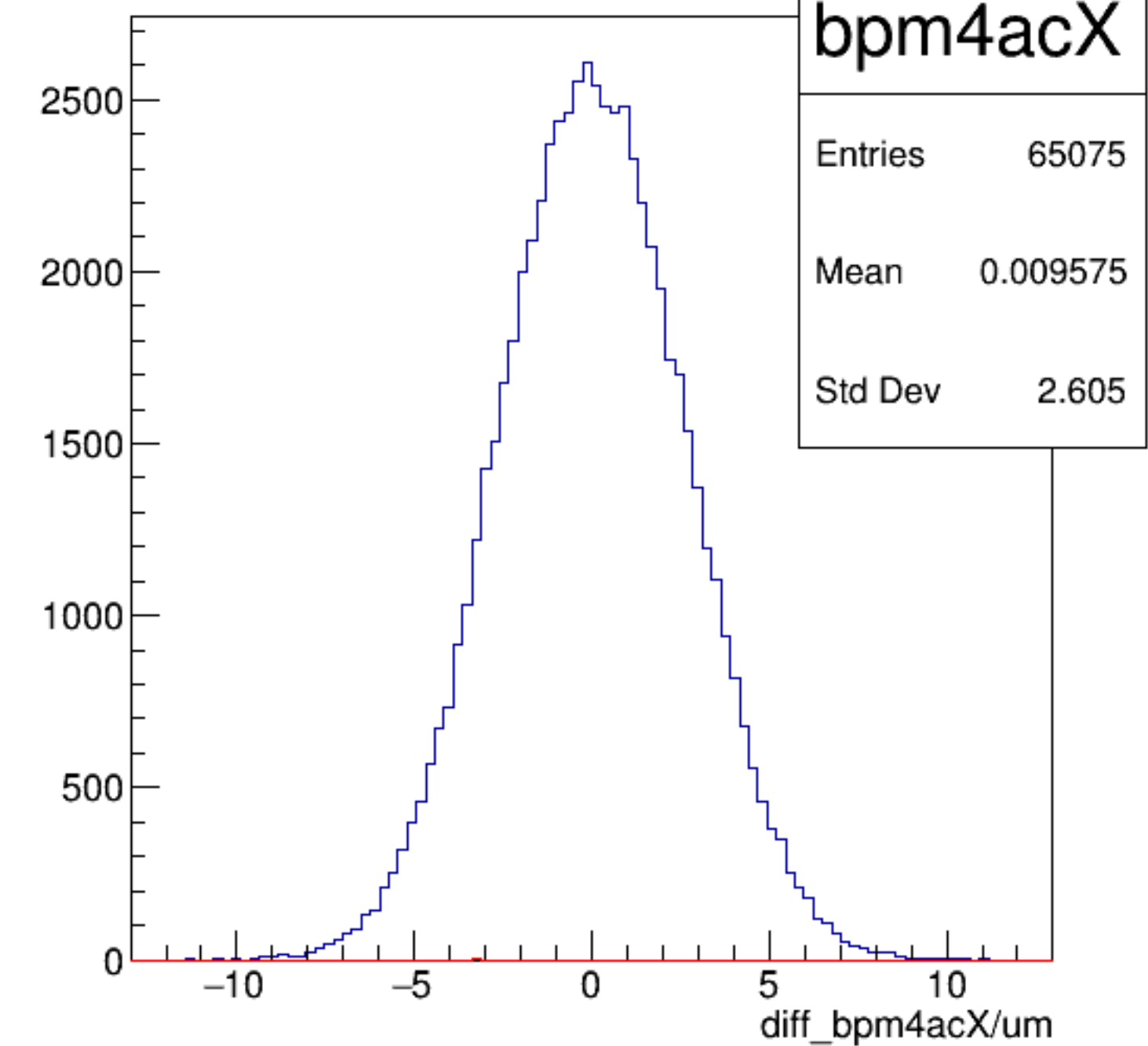
diff_bpm4acX/um {ErrorFlag==0}
