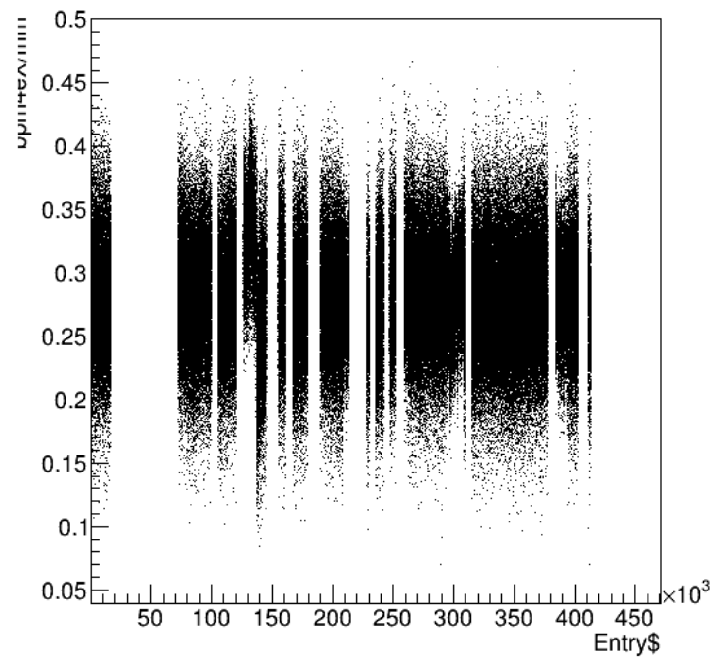
bpm4eX/mm:Entry$ {ErrorFlag==0}
