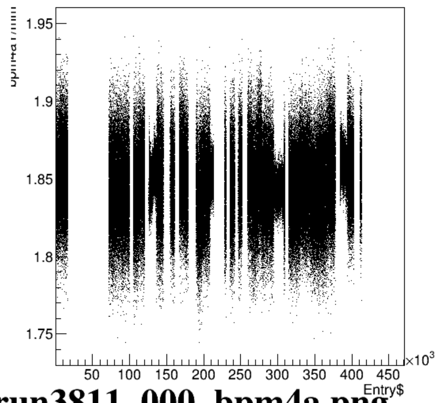
bpm4aY/mm:Entry$ {ErrorFlag==0}
