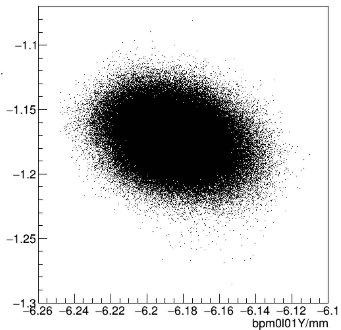
bpm0l01X/mm:bpm0l01Y/mm {ErrorFlag==0}
