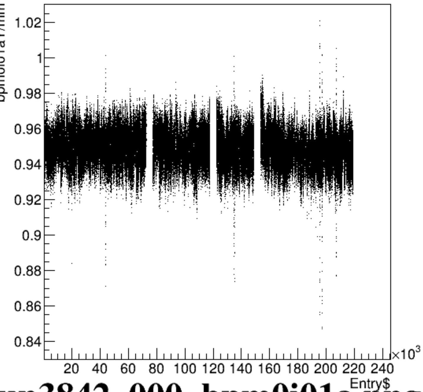
bpm0i01aY/mm:Entry$ {ErrorFlag==0}
