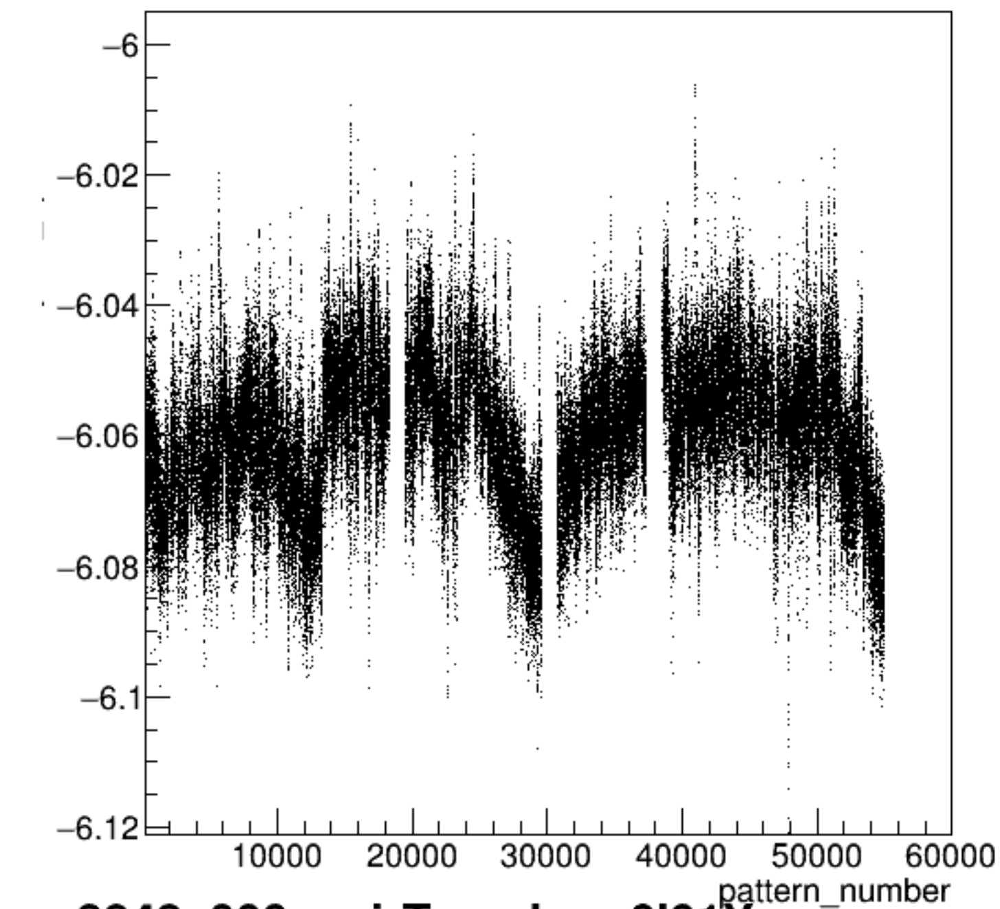
run3842_000_pairTree_bpm0l01Y.png
