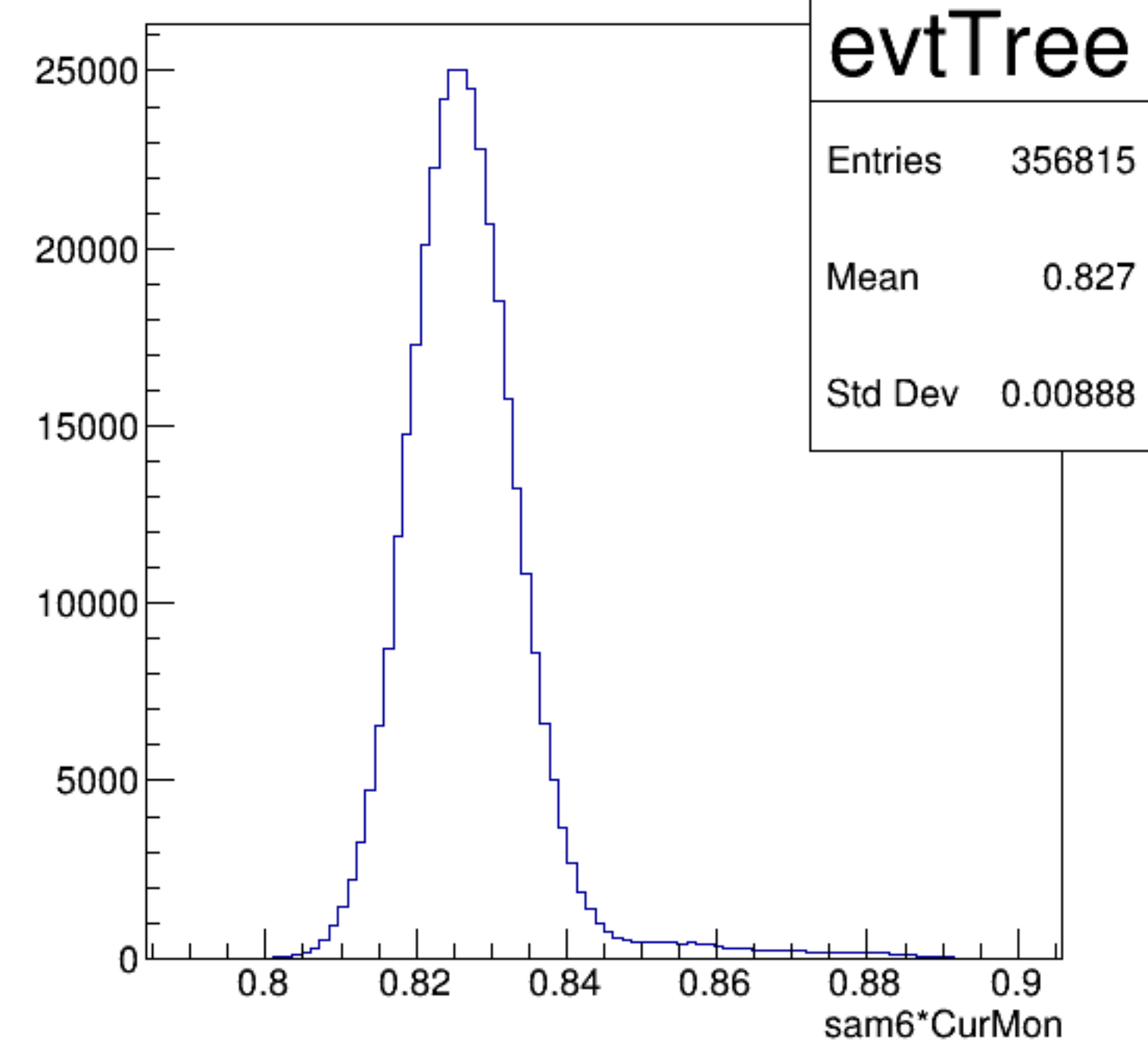
sam6*CurMon {ErrorFlag==0}
