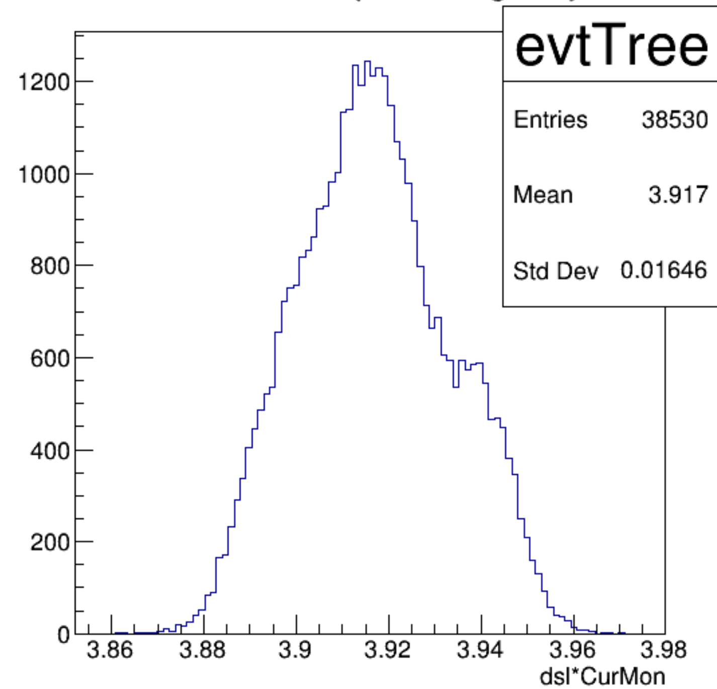
dsl*CurMon {ErrorFlag==0}
